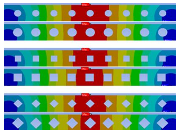
Gambar 8. Perubahan besaran defleksi balok pada berbagai dimensi dan bentuk bukaan balok.
