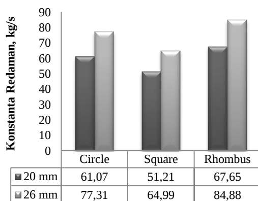
Gambar 10. Korelasi antara bentuk dan bukaan dan konstanta redaman
