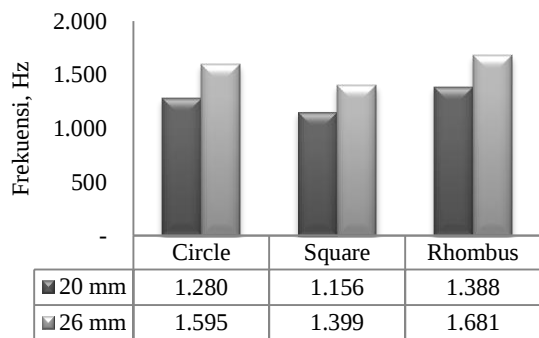
Gambar 9. Korelasi antara bentuk dan bukaan dan frekuensi balok.
