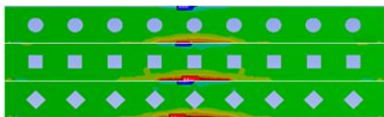
Gambar 6. Distribusi konsentrasi tegangan pada berbagai bukaan balok
