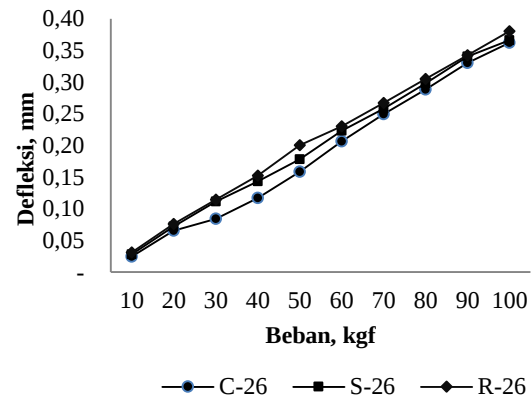
Gambar 7. Korelasi antara defleksi dan bentuk bukaan balok (a) dimensi 20mm, (b) 26 mm
