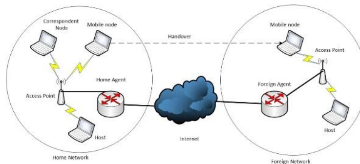
Gambar 2. Topologi Jaringan MIPv6
