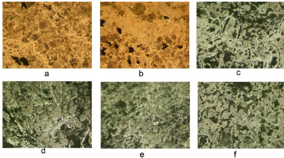
Figures 2 Optical microscope observation of MMC morphology with 100x magnification: (a). 20 vol.% Al 2 O 3 : 14 vol.% Mg (b). 20 vol.% Al 2 O 3 : 15 vol.% Mg (c). 20 vol.% Al 2 O 3 : 16 vol.% Mg (d). 10 vol.% Al 2 O 3 : 14 vol.% Mg (e). 20 vol.% Al 2 O 3 : 15 vol.% Mg (f). 10 vol.% Al 2 O 3 : 16 vol.% Mg.
