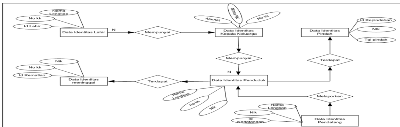
Gambar 8. Entity relationship diagram (ERD) penduduk Desa Sukamaju
