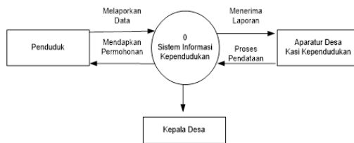
Gambar 1. Diagram konteks
