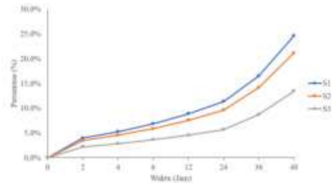
Gambar 4.3 Grafik Presentase Penyerapan Minyak
