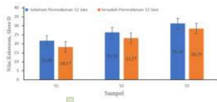
Gambar 4.5 Hasil Uji Kekerasan
