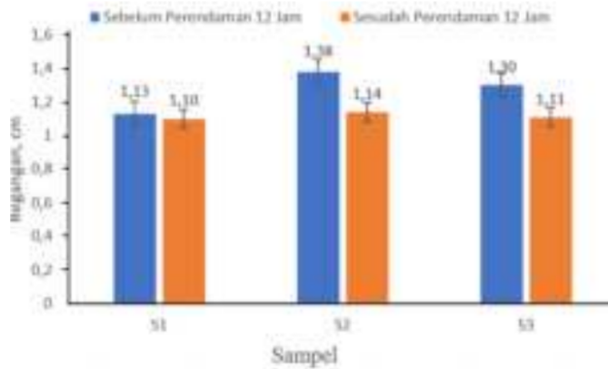
Gambar 4.8 Hasil Regangan
