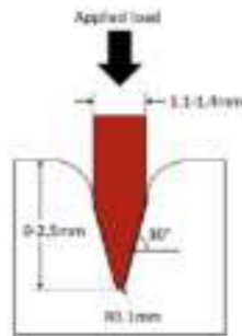
Gambar 2.10 Metode Pengujian Kekerasan Shore D [28]
