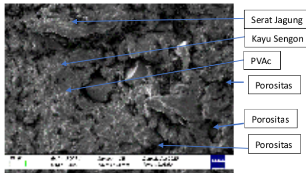
Gambar 4.9 Morfologi Permukaan Sampel S3
