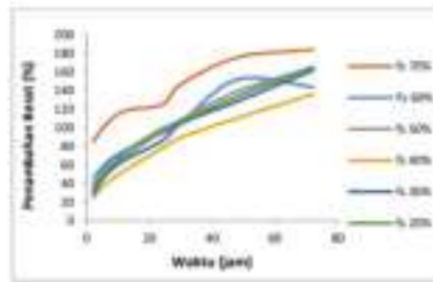
Gambar 2.1 Grafik penyerapan air pada komposit [5]
