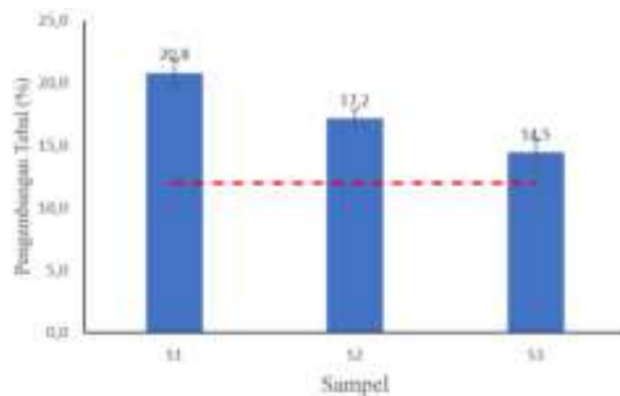
Gambar 4.2 Pengembangan Tebal
