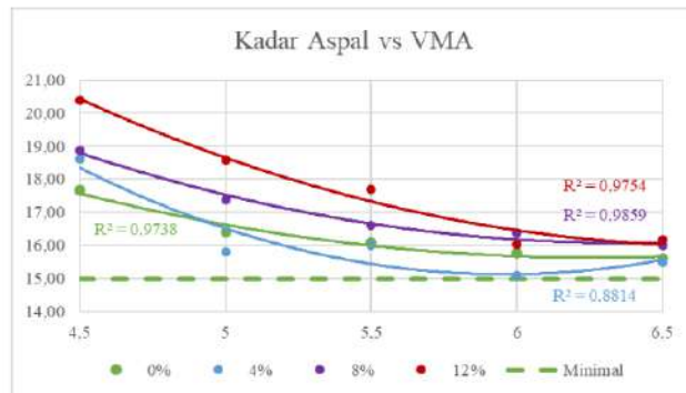
Gambar 5.18 Grafik perbandingan kadar aspal vs VMA
