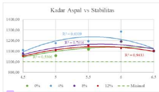
Gambar 5.20 Grafik perbandingan kadar aspal vs stabilitas (Sumber : Analisis penulis, 2025)
