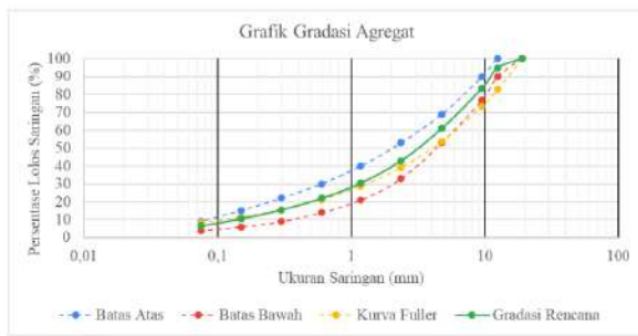
Gambar 4.5 Grafik gradasi agregat beraspal lapis aus (AC-WC)
