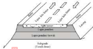
Gambar 3.2 Struktur perkerasan kaku
