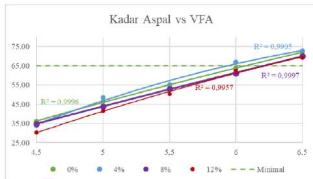
Gambar 5.19 Grafik perbandingan kadar aspal vs VFA
