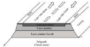
Gambar 3.1 Struktur perkerasan lentur
