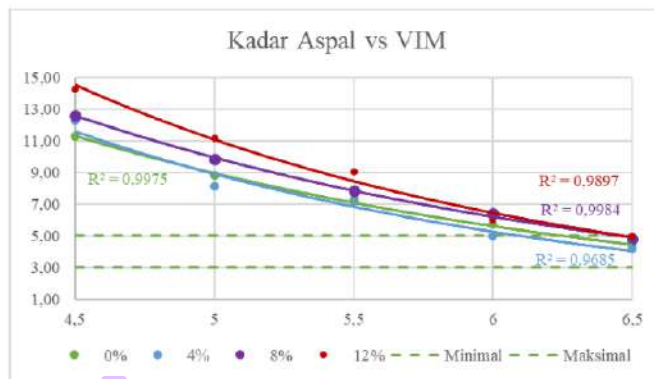
Gambar 5.17 Grafik perbandingan kadar aspal vs VIM
