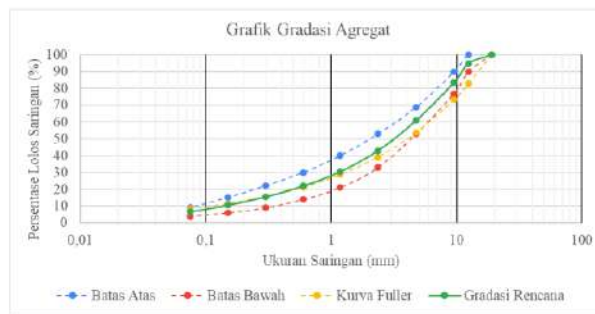
Gambar 5.14 Grafik gradasi agregat beraspal lapis aus (AC-WC)
