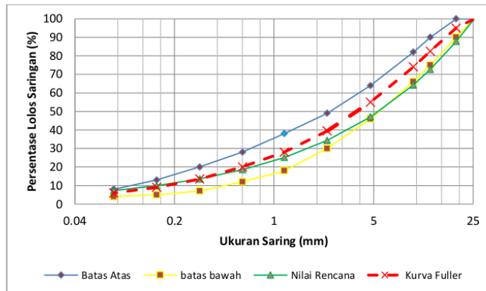
Gambar 5.20 Grafik Gradasi Campuran Aspal Lapis AC-BC
