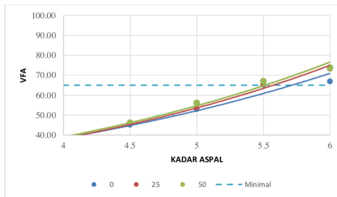
Gambar 5.25 Grafik Hubungan Nilai VFA dan Kadar Aspal
