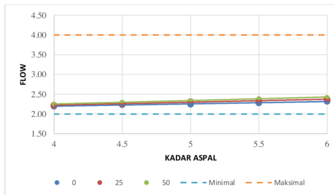
Gambar 5.27 Hubungan Nilai Flow dan Kadar Aspal
