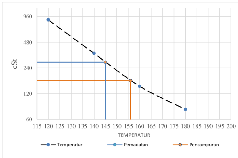
Gambar 5.12 Grafik Pengujian Viskositas
