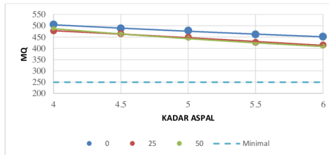
Gambar 5.28 Hubungan Nilai MQ dan Kadar Aspal
