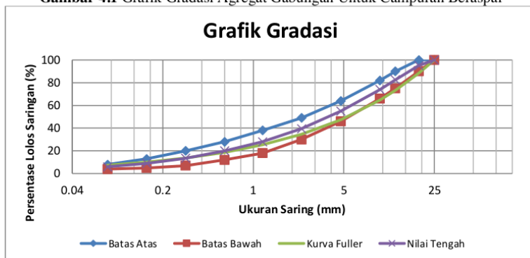
Gambar 4.1 Grafik Gradasi Agregat Gabungan Untuk Campuran Beraspal
