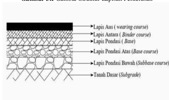
Gambar 3.1 Gambar Struktur Lapisan Perkerasan
