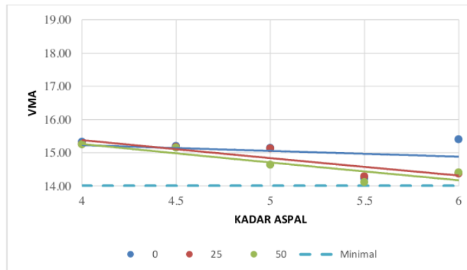
Gambar 5.23 Grafik Hubungan Nilai VMA dan Kadar Aspal
