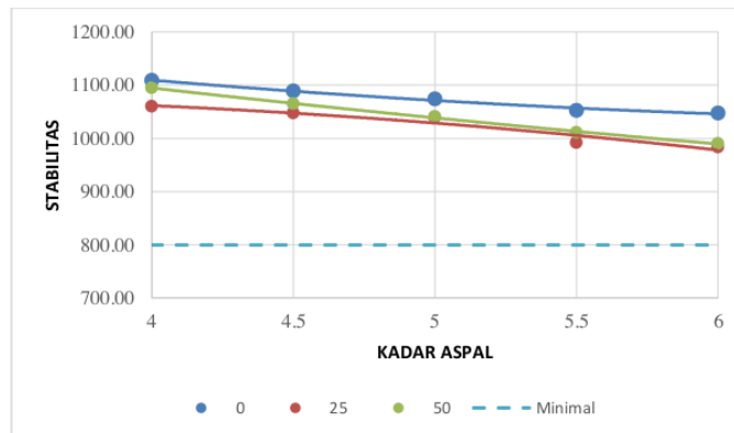
Gambar 5.26 Hubungan Nilai Stabilitas dan Kadar Aspal
