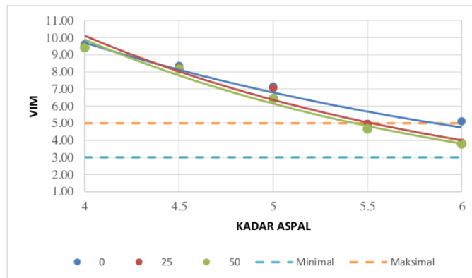
Gambar 5.24 Grafik Hubungan Nilai VIM dan Kadar Aspal
