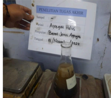
Gambar 5.5 Pengujian Berat Jenis Agregat Halus
