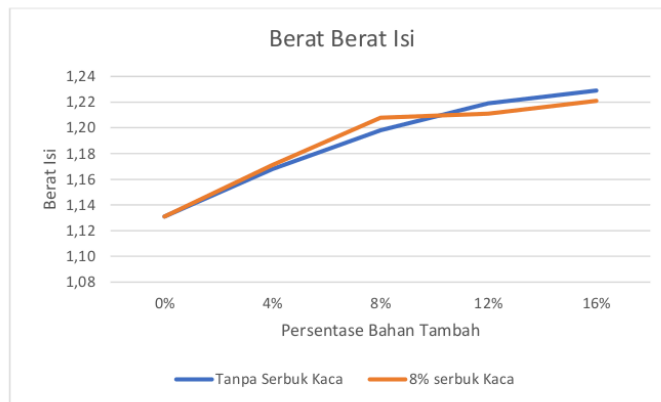
Gambar 5.20 Grafik Perbandingan Berat Isi dengan Persentase Bahan Tambah (Sumber : Data Penulis, 2023)
