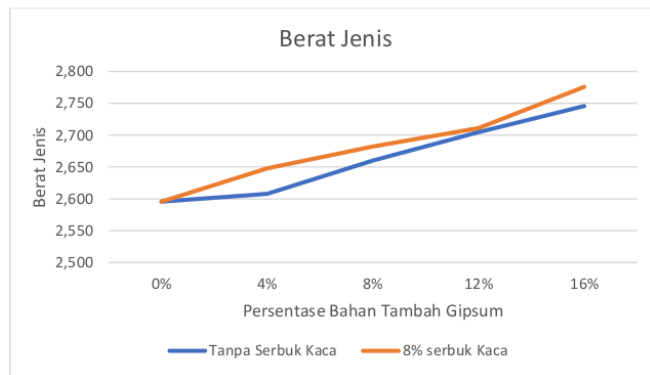
Gambar 5.19 Grafik Berat Jenis Terhadap Setiap Persentase Bahan Tambah
