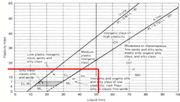
Gambar 5.10 Grafik Hubungan Batas Cair dan Indeks Plastisitas
