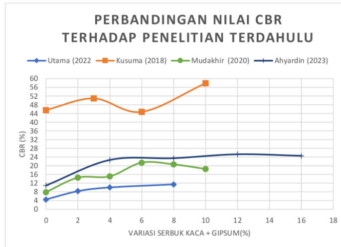
Gambar 5.27 Grafik Hasil CBR dengan Penelitian Terdahulu
