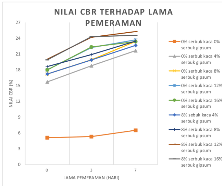
Gambar 5.26 Grafik Hasil CBR
