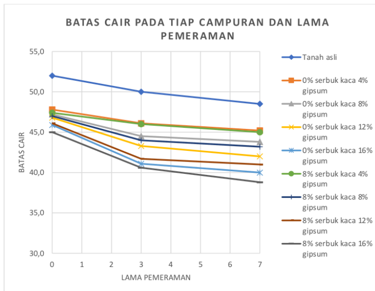
Gambar 5.21 Grafik Batas Cair Terhadap Lama Pemeraman
