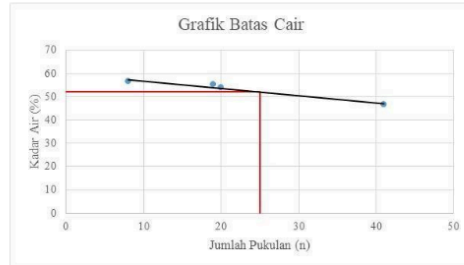
Gambar 5.8 Grafik Hubungan Kadar Air dengan Jumlah Ketukan
