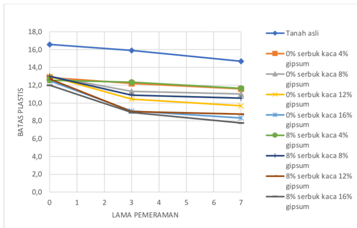
Gambar 5.23 Grafik Indeks Plastisitas Terhadap Lama Pemeraman
