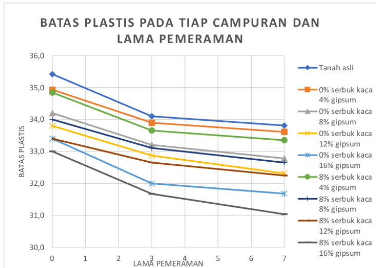
Gambar 5.22 Grafik Batas Plastis Terhadap Lama Pemeraman
