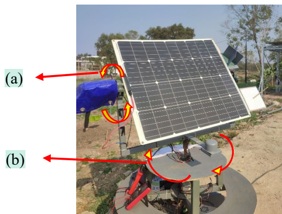
Gambar 4.1 Visualisasi solar tracking dual axis system , (a) Rotasi sudut altitude sebesar 270^\circ , (b) Rotasi sudut azimuth sebesar 360^\circ
