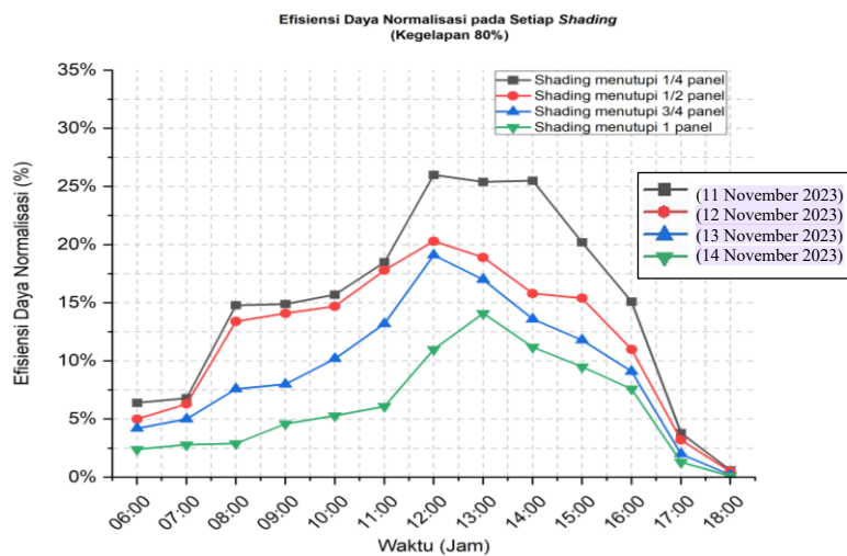
Gambar 4.30 Grafik Efisiensi Daya Normalisasi Shading 80%
