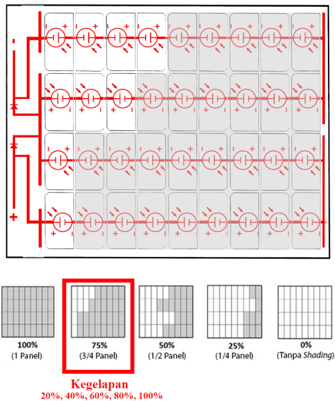
Gambar B.4 Rangkaian pada penutupan \frac{3}{4} panel
