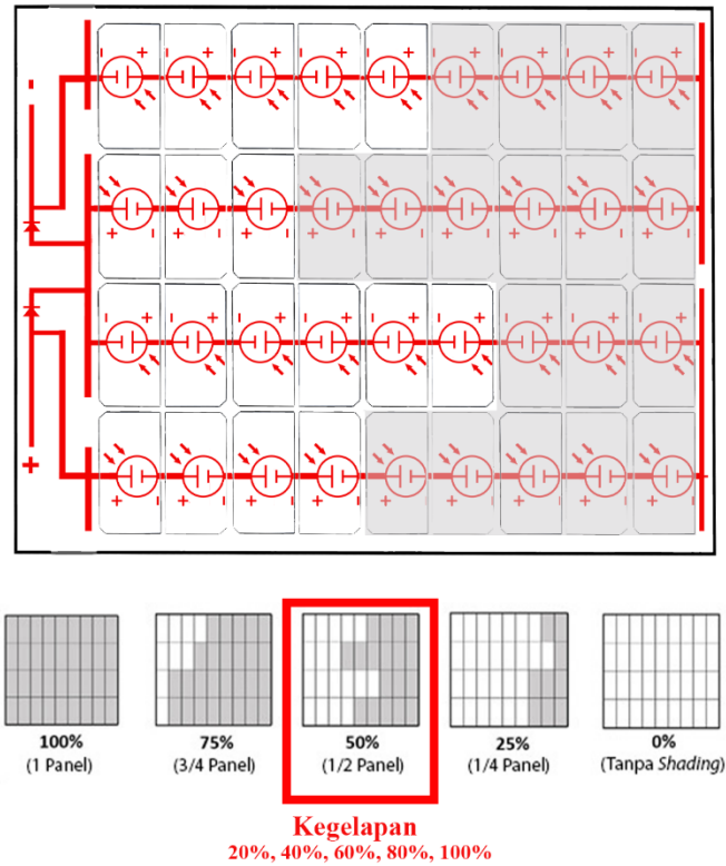
Gambar B.3 Rangkaian pada penutupan \frac{1}{2} panel
