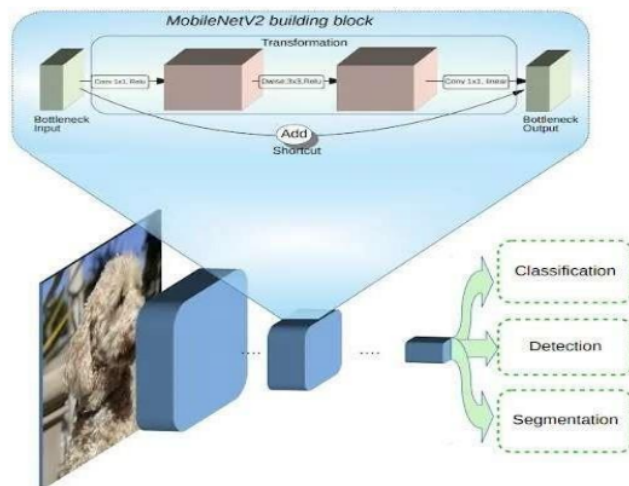
Gambar 2.7 Tahapan MobileNetV2 [44]
