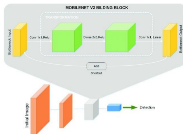
Gambar 2.8 Arsitektur MobileNetV2 [41]
