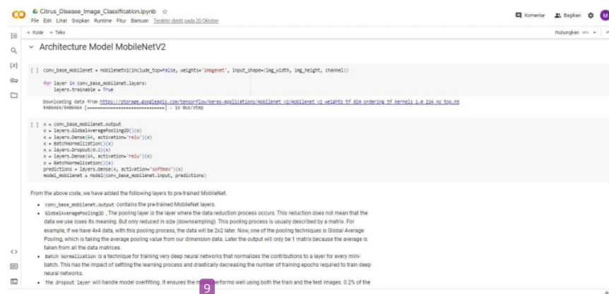
Gambar 4.2 Arsitektur MobilenetV2
