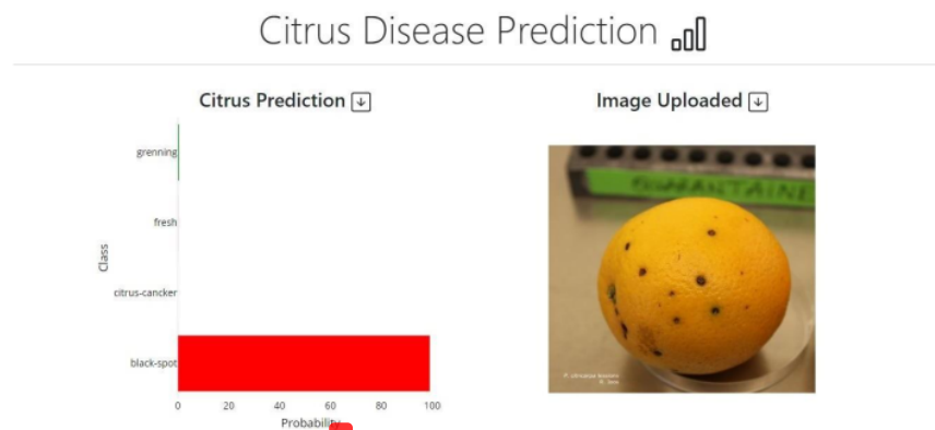
Gambar 4.12 Hasil Deteksi
