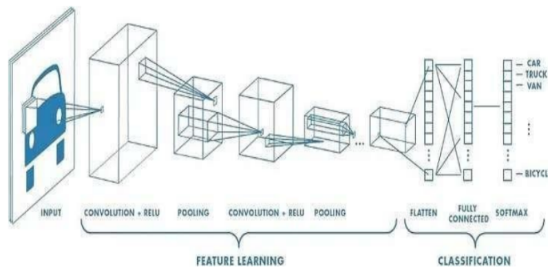
Gambar 2.6 Tahapan CNN [39]
