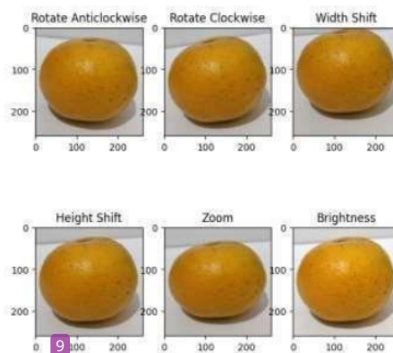
Gambar 3.3 Augmentasi Data
