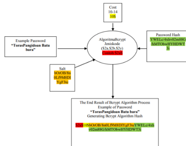
Gambar 2.2 Proses Keamanan Kata Sandi dengan Bcrypt [33]
