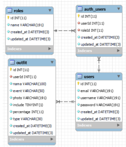
Gambar 4.8 Perancangan Basis Data Aplikasi
