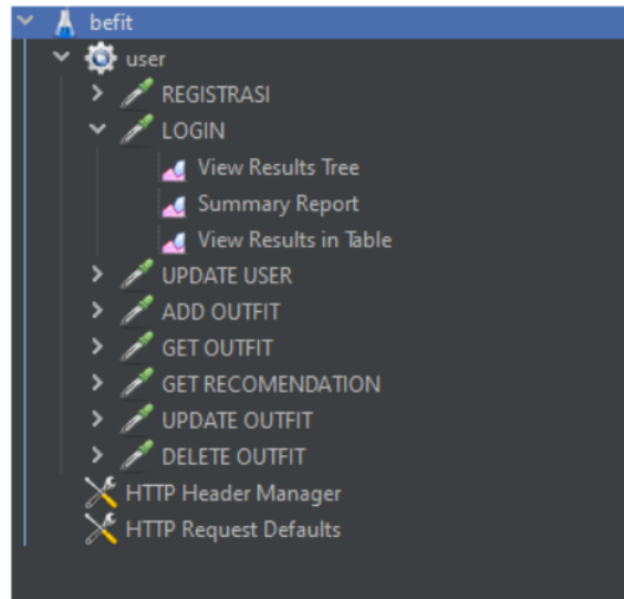
Gambar B. 1 Testing Plan API dengan Jmeter
