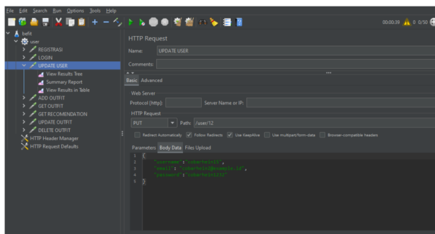
Gambar B. 4 Pengujian API Update User
