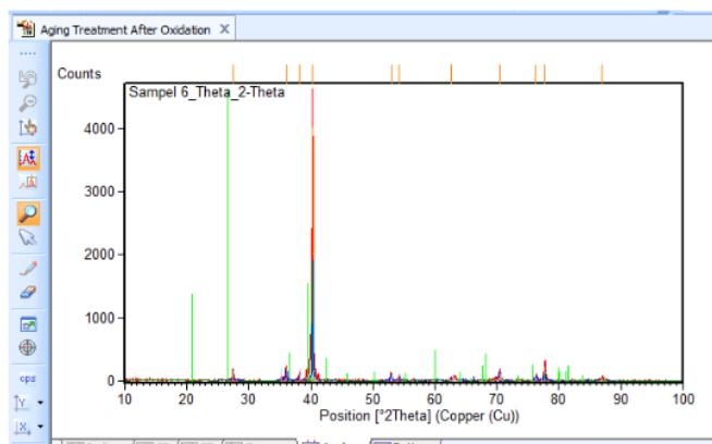
Gambar B.15 XRD Sampel Aging Treatment Setelah Uji Oksidasi
