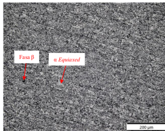
9 Gambar 4.4 Struktur Mikro As-Cast Paduan Ti-6Al-4V
