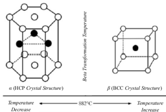
Gambar 2.1 Struktur Kristal Titanium [24].
