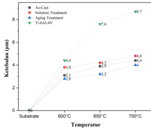
Gambar 4.13 Grafik Ketebalan Lapisan Oksida Setiap Sampel
