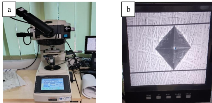
Gambar 3.7 a) Mesin Kekerasan Vickers , b) Area Pembebanan
