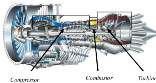
Gambar 2.4 Mesin Turbin Jet [34].
