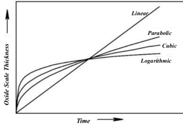
Gambar 2.12 Variasi laju reaksi oksidasi [42].
