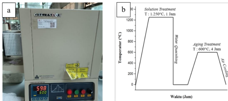
Gambar 3.4 a) Tube Furnace , b) Skema Perlakuan Panas
