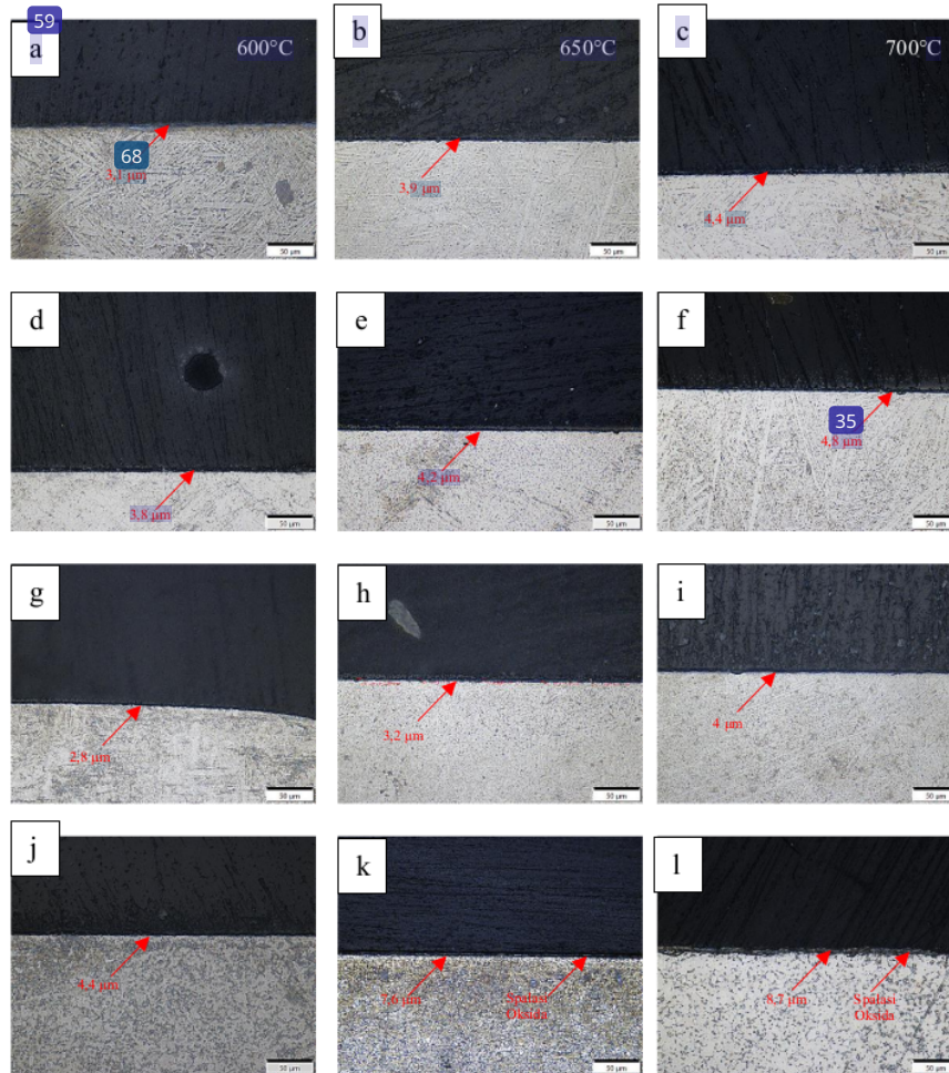
Gambar 4.12 Pengamatan Mikroskop Optik Setelah Pengujian Oksidasi. (a)-(c)
