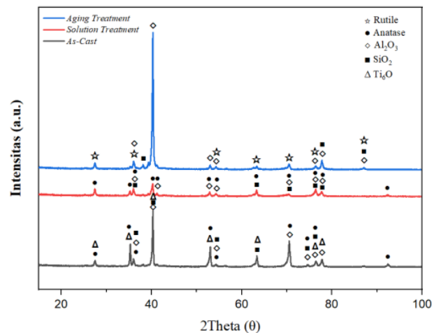
Gambar 4.14 Data XRD Setelah Pengujian Oksidasi 700°C
