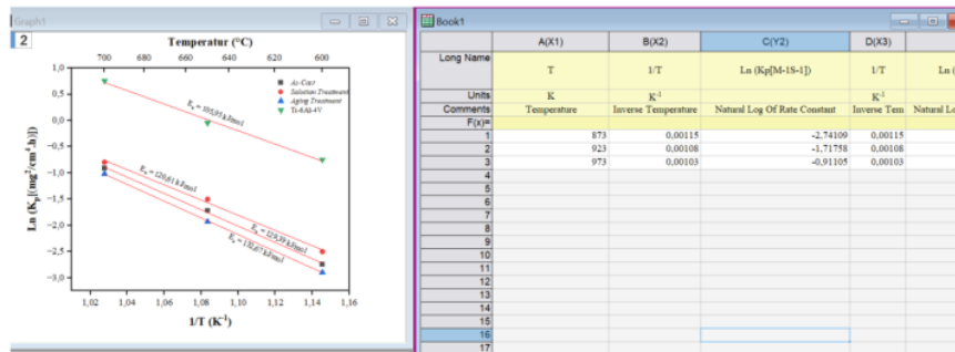
Gambar B.12 Data Hasil Plot Arhenius Oksidasi
