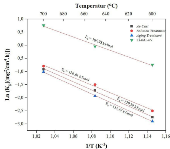
Gambar 4.9 Plot Arrhenius Oksidasi
