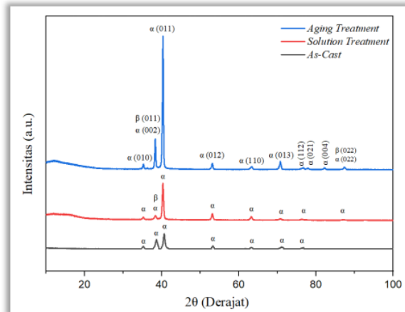
Gambar 4.6 Hasil Analisis XRD Dengan Perbedaan Sampel
