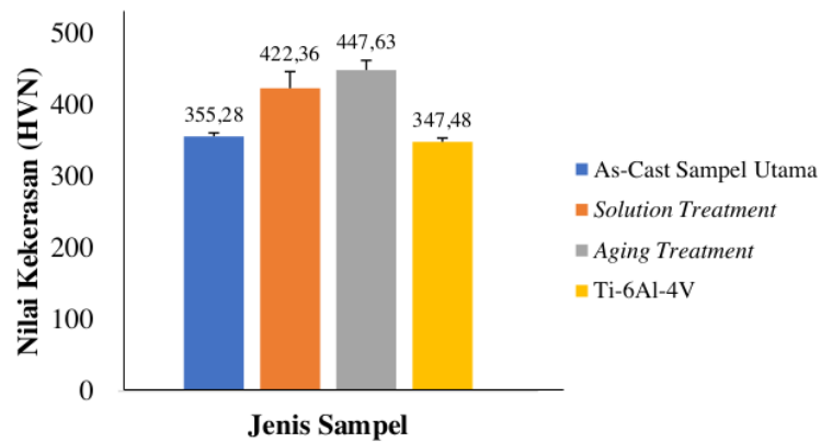
Gambar 4.7 Nilai Kekerasan Paduan Ti-6Al-5Nb-3Sn-1Zr-0,5Si dan Ti-6Al-4V
