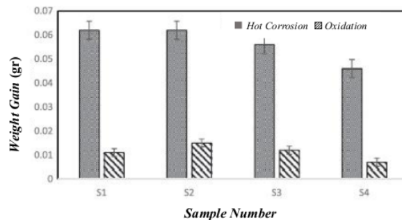
Gambar 2.11 Perbandingan Berbagai Sampel Dengan Pertambahan Berat [17].
