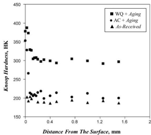
Gambar 2.10 Nilai Kekerasan Dengan Perbedaan Perlakuan Panas [41]
