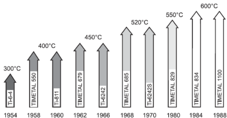
Gambar 2.3 Peningkatan Temperatur Titanium Paduan [32].
