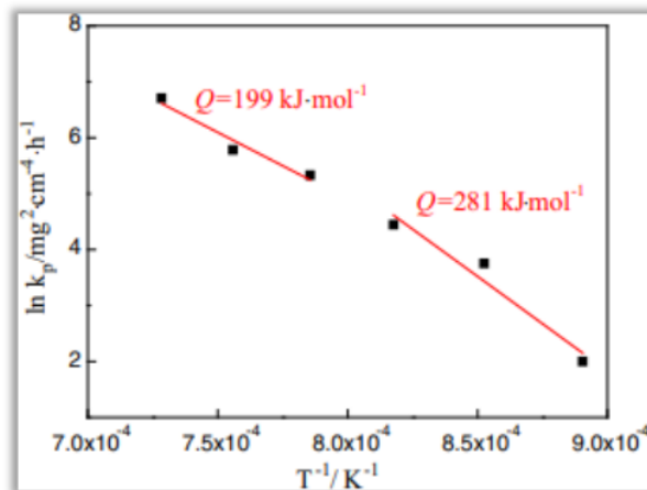
Gambar 2.13 Kurva Arrhenius Konstanta Laju Parabola K_p Ti-6Al-4V [44].
