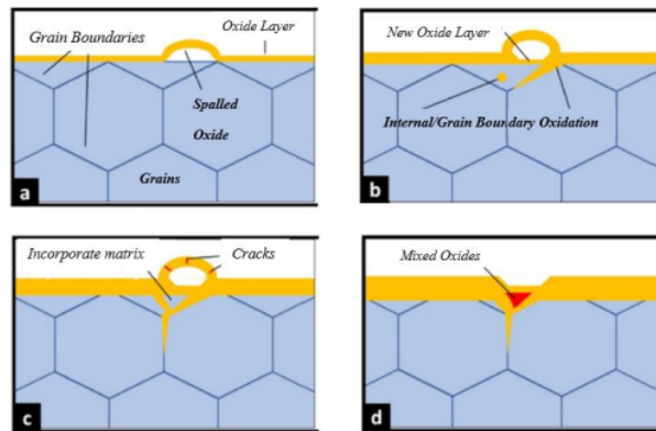
Gambar 4.10 Mekanisme Oksidasi Pada Batas Butir [67].
