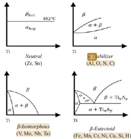
Gambar 2.2 Pengaruh Unsur Paduan Pada Titanium [26].
