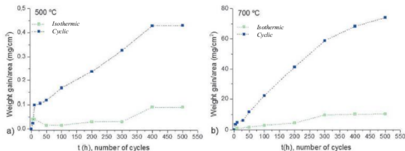
Gambar 2.14 Uji Oksidasi Siklik Ti-6Al-4V [9].
