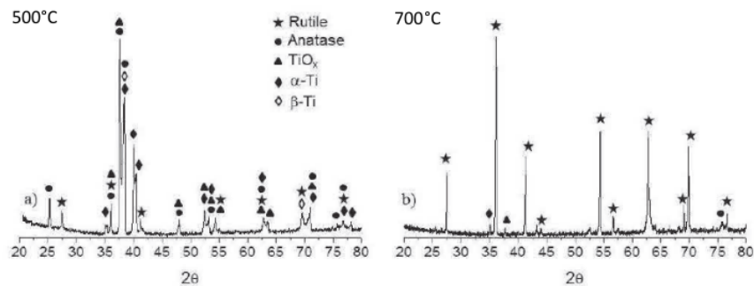
Gambar 2.15 Hasil Uji XRD Setelah Uji Oksidasi Siklik [9].
