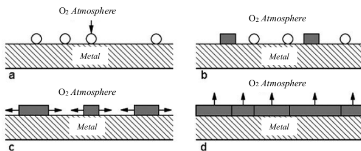
Gambar 2.6 Skematik Proses Oksidasi Titanium [37].
