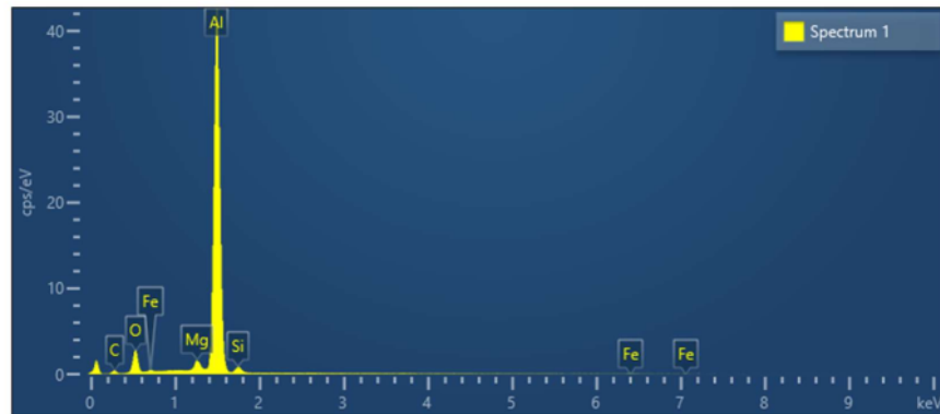
Gambar 4.25 Spektrum EDS Sampel dengan Reduksi 5%
