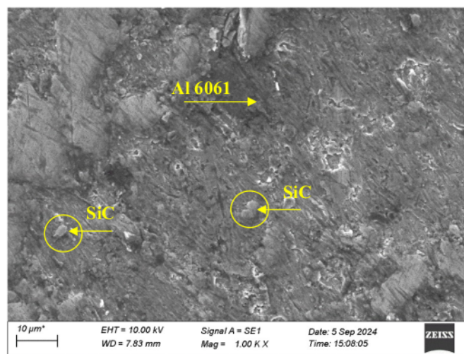
Gambar 4.8 Sampel Komposit dengan Reduksi Ketebalan 2%
