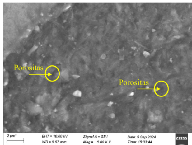
Gambar 4.12 Cacat pada Sampel dengan Reduksi 4%
