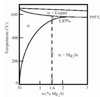
Gambar 2.2 Diagram Fasa Al 6061
