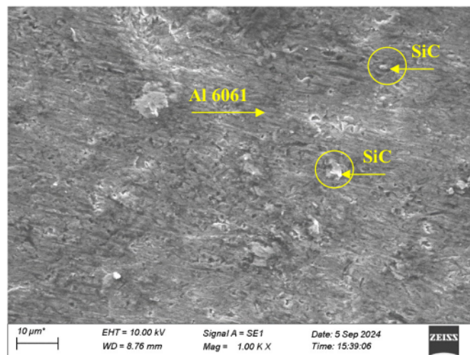
Gambar 4.10 Sampel Komposit dengan Reduksi Ketebalan 5%
