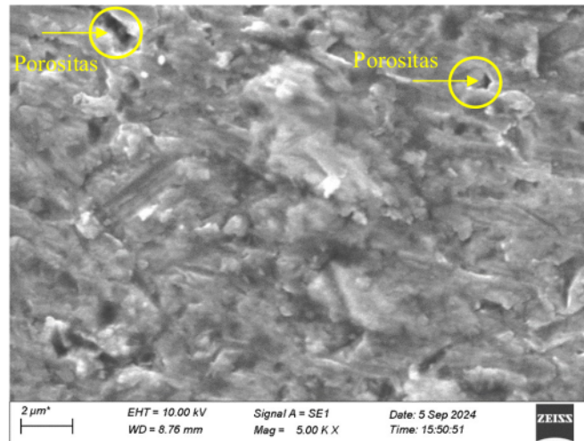
Gambar 4.13 Cacat pada Sampel dengan Reduksi 5%
