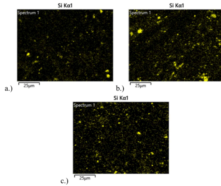
Gambar 4.20 Unsur Si pada Komposit (a. Reduksi 2%; b. Reduksi 4%; c. Reduksi 5%)
