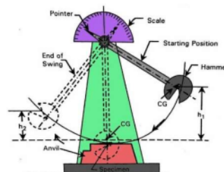
Gambar 2.7 Uji Impak (Sumber: anakteknik.co.id)
