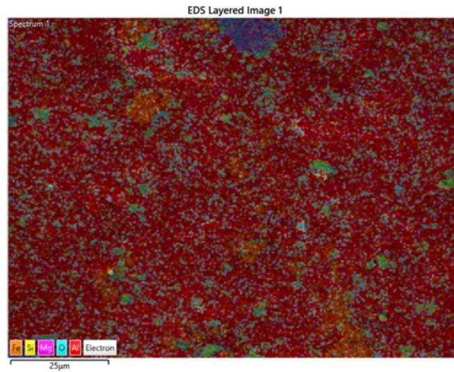
Gambar 4.16 EDS Mapping Sampel Komposit Hasil Reduksi 5%
