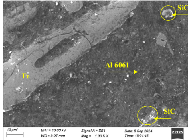
Gambar 4.9 Sampel Komposit dengan Reduksi Ketebalan 4%
