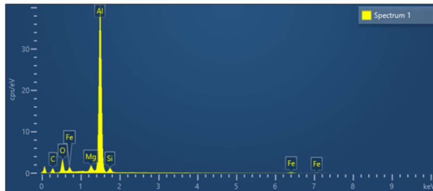
Gambar 4.24 Spektrum EDS Sampel dengan Reduksi 4%
