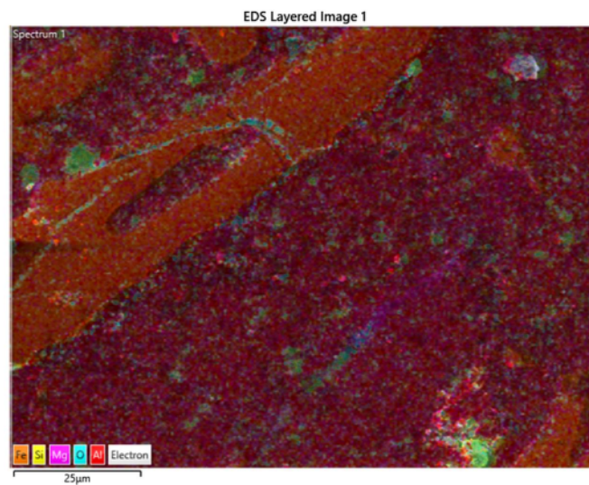
Gambar 4.15 EDS Mapping Sampel Komposit Hasil Reduksi 4%
