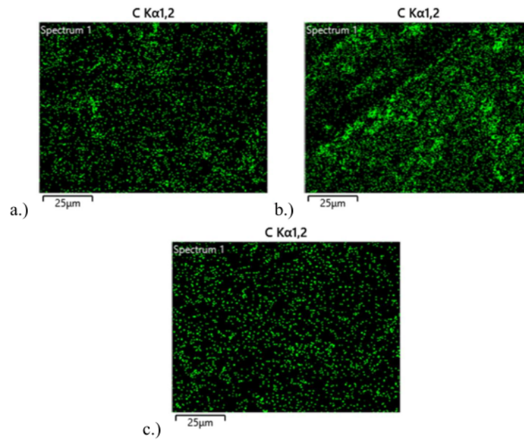
Gambar 4.22 Unsur C pada Komposit (a. Reduksi 2%; b. Reduksi 4%; c. Reduksi 5%)
