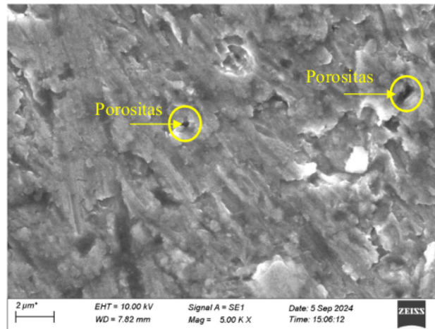
Gambar 4.11 Cacat pada Sampel dengan Reduksi 2%
