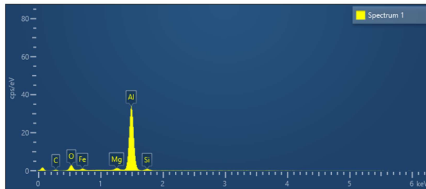
Gambar 4.23 Spektrum EDS Sampel dengan Reduksi 2%
