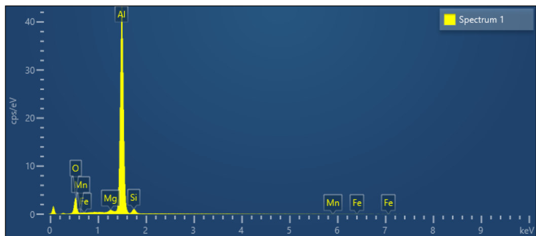
Figure 2. Al 6061 + Al 2 O 3 5%
