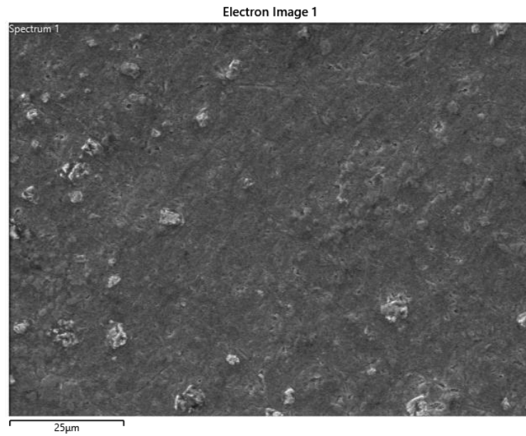
Figure 1. Al 6061 + Al 2 O 3 10%
