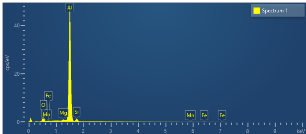
Figure 3. Al 6061 + Al 2 O 3 15%
