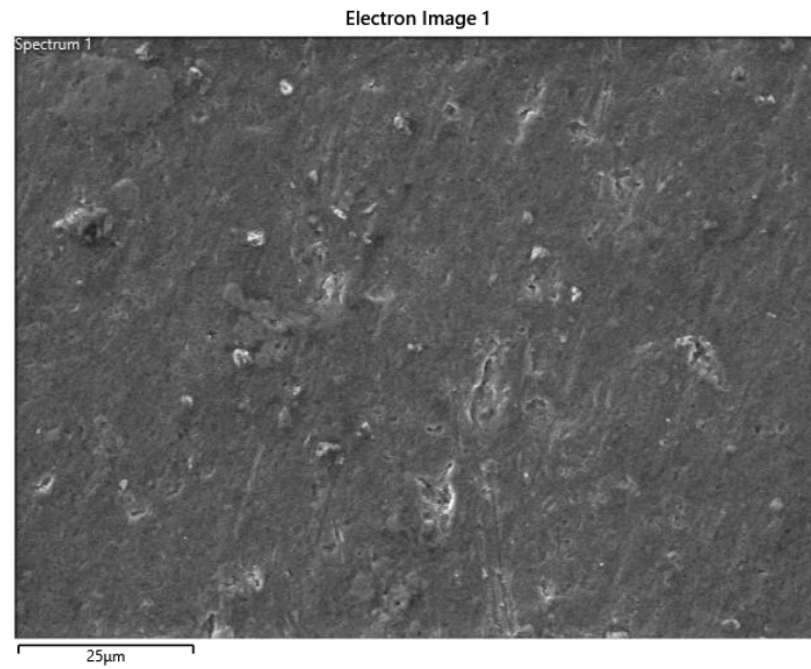
Figure 3. Al 6061 + Al 2 O 3 15%
