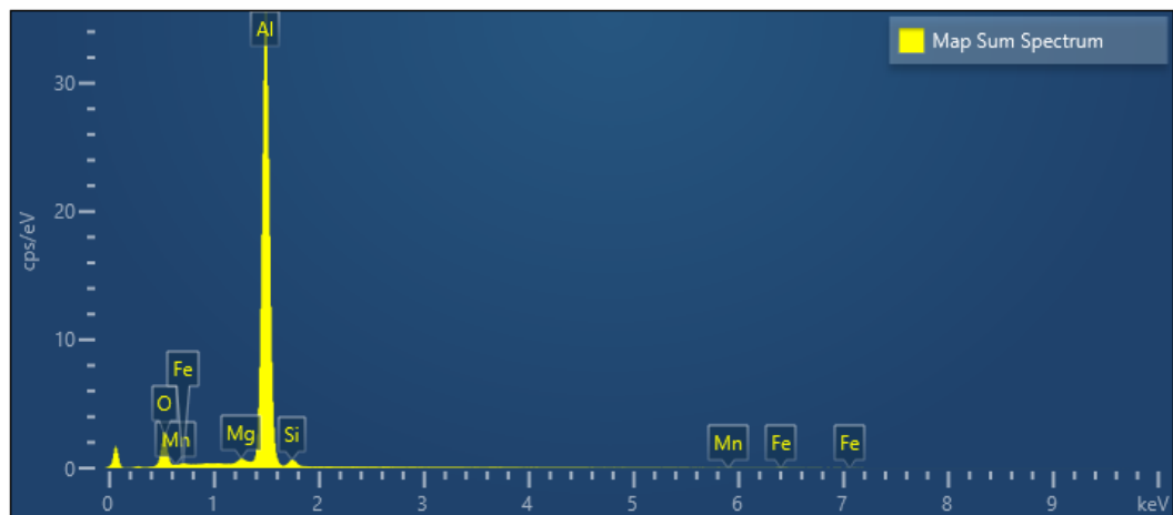
Figure 1. Al 6061 + Al 2 O 3 10%
