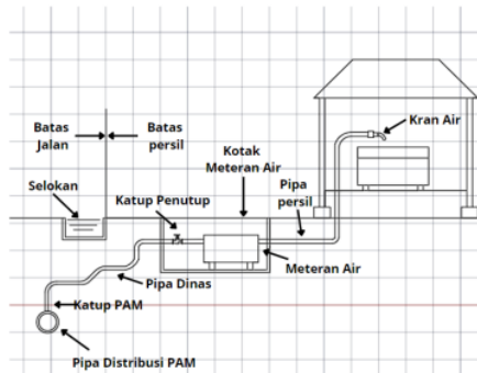
Gambar 2.1 Sistem Sambungan Langsung
