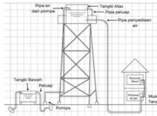
Gambar 2.2 Sistem Tangki Atas
