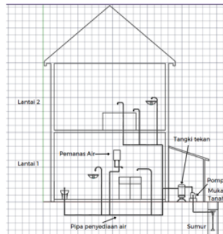
Gambar 2.3 Sistem Tangki Tekan
