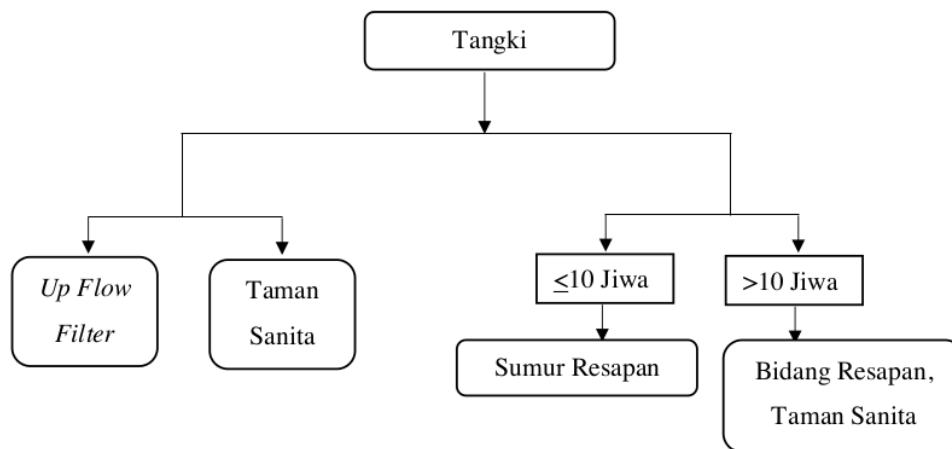
Gambar 2.4 Diagram Pengolahan Lanjutan Air Keluar (Sumber : SNI 2398-2017)
