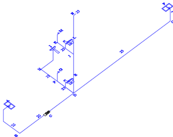
Gambar 4.3 Isometri Pipa Air Bersih
