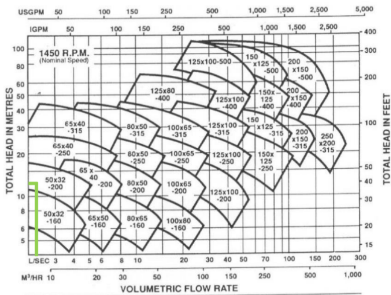
Gambar 4.6 Grafik Pompa Sentrifugal Grundfos
