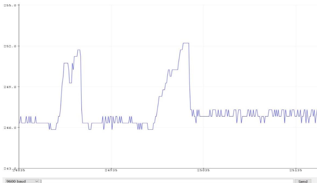
Gambar 2 Sampel pengujian 4 ampere
