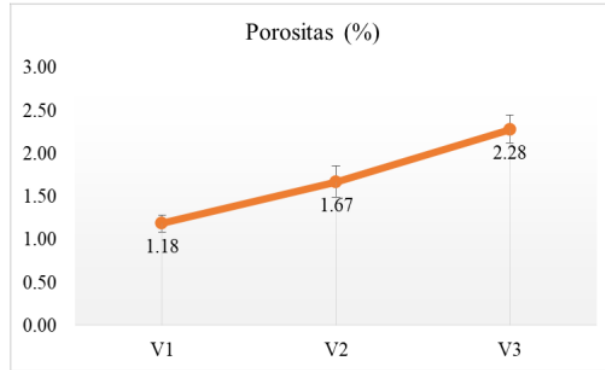
Gambar 4.2 Grafik Nilai Porositas
