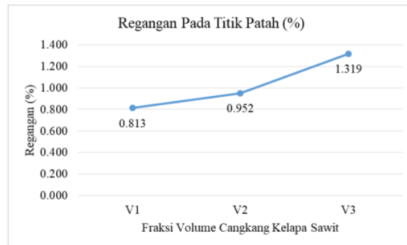
Gambar 4.6 Grafik Regangan Terhadap Fraksi Volume
