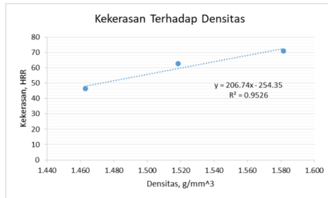
Gambar 4.10 Grafik Hubungan Kekerasan dan Densitas
