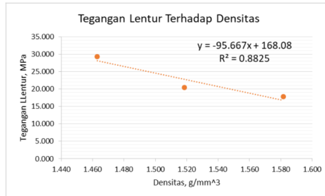
Gambar 4.9 Grafik Hubungan Kekuatan Lentur dan Densitas
