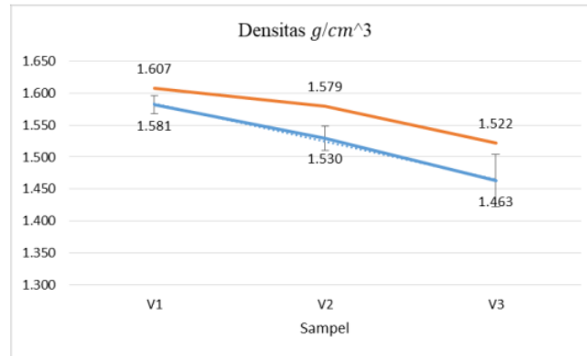
Gambar 4.1 Grafik Nilai Densitas Aktual dan Teoritis
