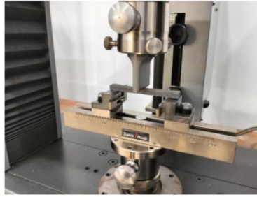
Gambar 3.2 Mesin Uji Lentur
