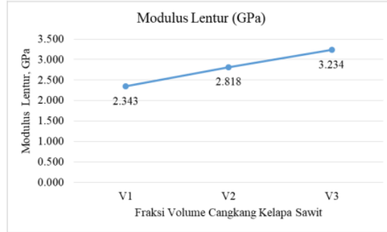
Gambar 4.5 Grafik modulus lentur Terhadap Fraksi Volume
