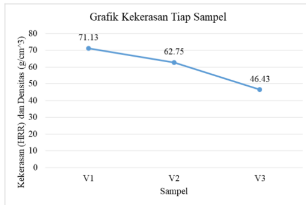
Gambar 4.12 Pengujian Kekerasan
