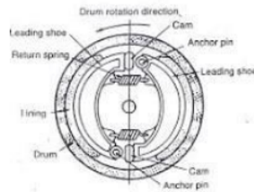
Gambar 2.1 Rem Tromol (Sumber : carmudi.co.id)
