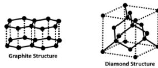
Gambar 2.6 Struktur Graphite
