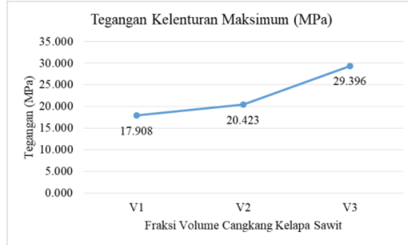
Gambar 4.7 Grafik Tegangan Lentur Maks Terhadap Fraksi Volume
