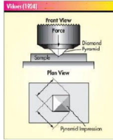
Gambar 2.5 Pengujian Vickers (Sumber : (Simanjong dkk., 2017))
