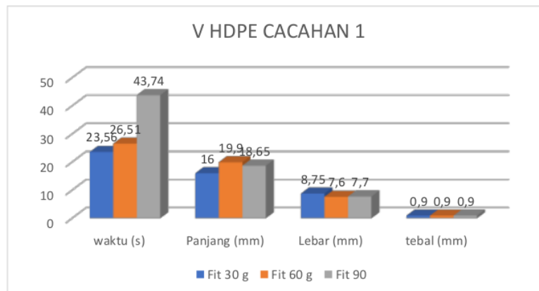
Gambar 4.8 Grafik V HDPE Cacahan 1
