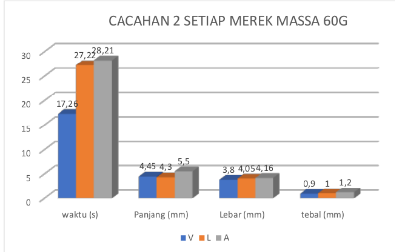
Gambar 4.17 Grafik Cacahan 2 Setiap Merek Massa 60g
