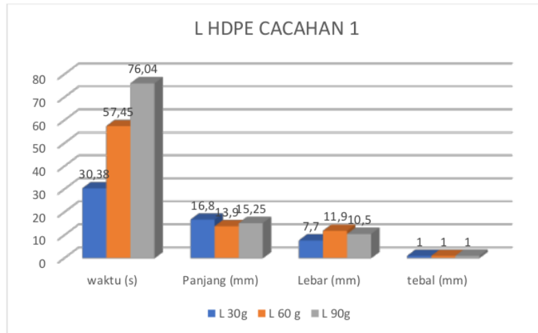
Gambar 4.10 Grafik L HDPE Cacahan 1
