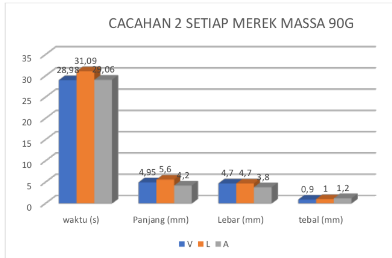
Gambar 4.19 Grafik Cacahan 2 Setiap Merek Massa 90g
