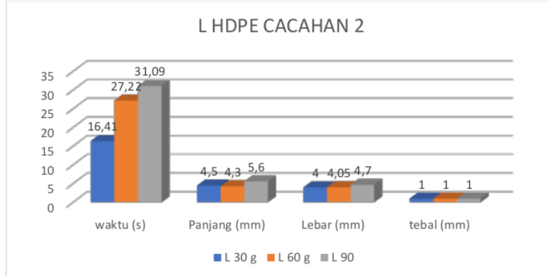
Gambar 4.11 Grafik L HDPE Cacahan 2
