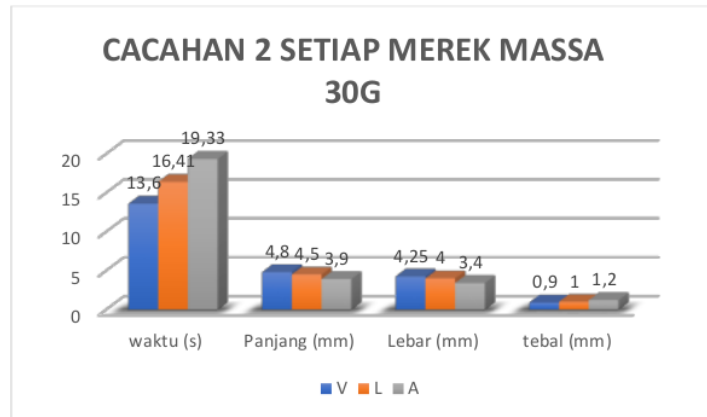
Gambar 4.15 Grafik Cacahan 2 Setiap Merek Massa 30g
