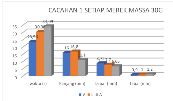
Gambar 4.14 Grafik Cacahan 1 Setiap Merek Massa 30g
