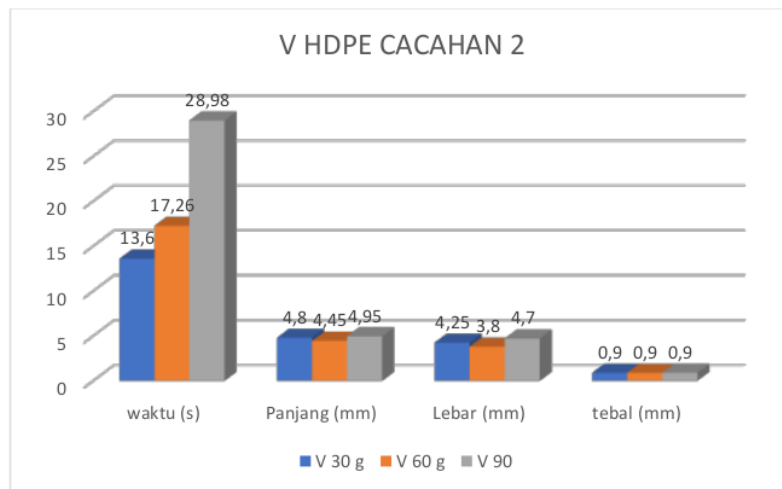
Gambar 4.9 Grafik V HDPE Cacahan 2
