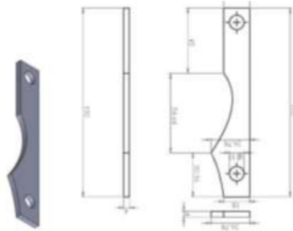
Gambar 3.8 Desain Mata Pisau
