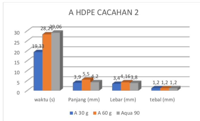
Gambar 4.13 Grafik A HDPE Cacahan 2
