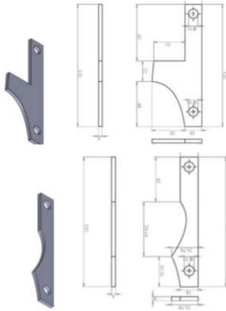
Gambar 4.4 Desain Mata Potong
