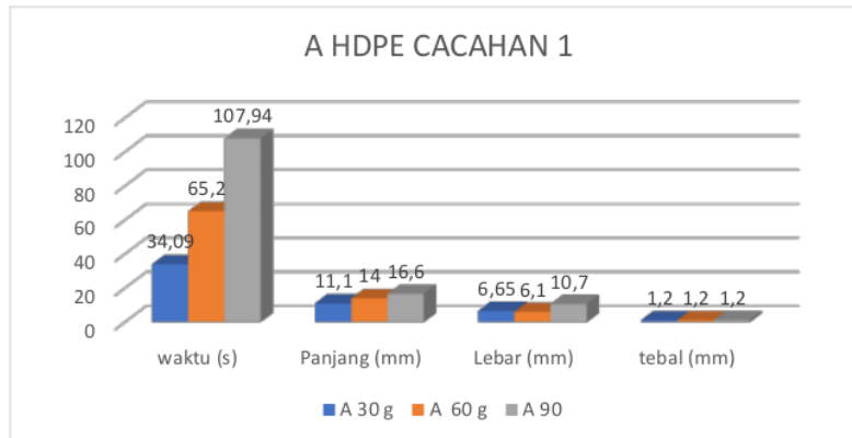
Gambar 4.12 Grafik A HDPE Cacahan 1
