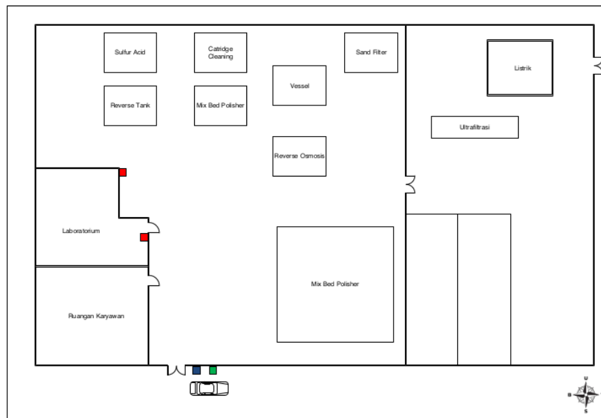
Gambar 7 Layout Gedung lantai 1
