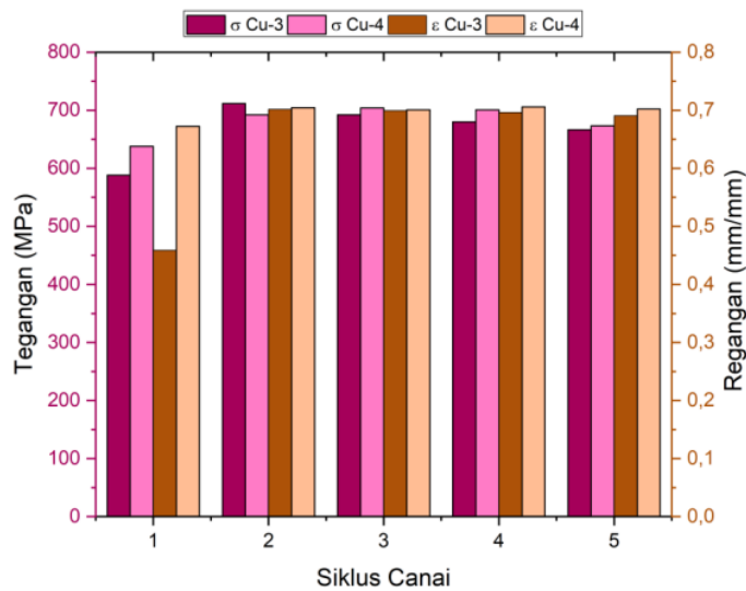
Gambar 4.16 Grafik Tegangan-Regangan Pelat Cu 3 Lapis dan 4 Lapis
