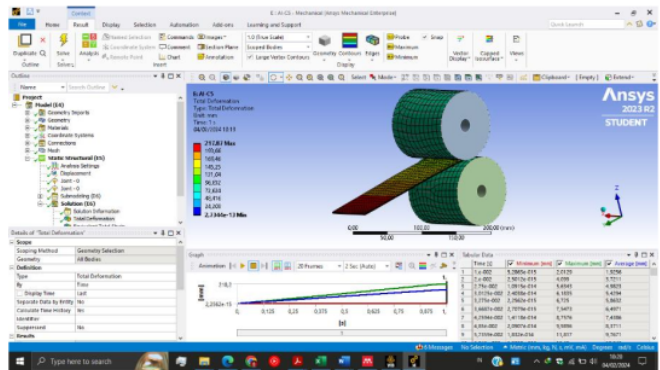
Gambar B.10 Hasil Simulasi Pencanaian Aluminium Empat Lapis
