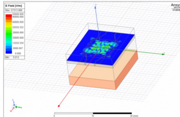
Gambar 4.20 Hasil Simulasi Radiasi dengan Tembaga Tiga Lapis
