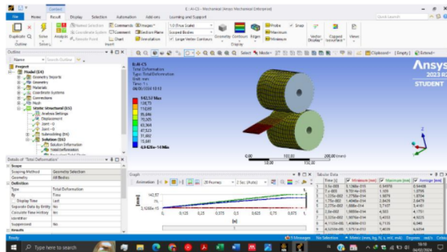
Gambar B.7 Hasil Simulasi Pencanaan Aluminium Tiga Lapis
