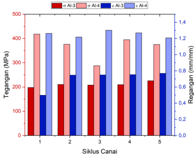
Gambar 4.15 Grafik Tegangan-Regangan Pelat Al 3 Lapis dan 4 Lapis
