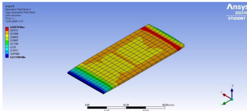
Gambar 4.10 Hasil Pencapaian Tembaga Tiga Lapis (a) Stress (b) Strain
