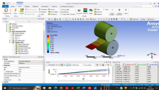
Gambar B.9 Hasil Simulasi Pencanaian Timbal Tiga Lapis
