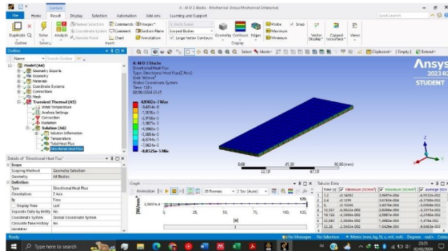
Gambar B.1 Hasil Simulasi Pemanasan Aluminium Tiga Lapis
