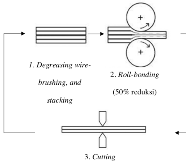
Gambar 2.6 Skema Siklus ARB [39]
