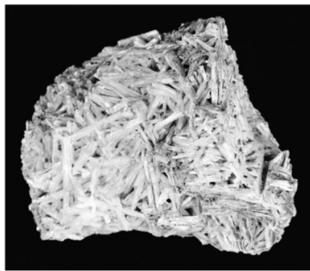
Gambar 2.4 Bijih Kerisit [21]
