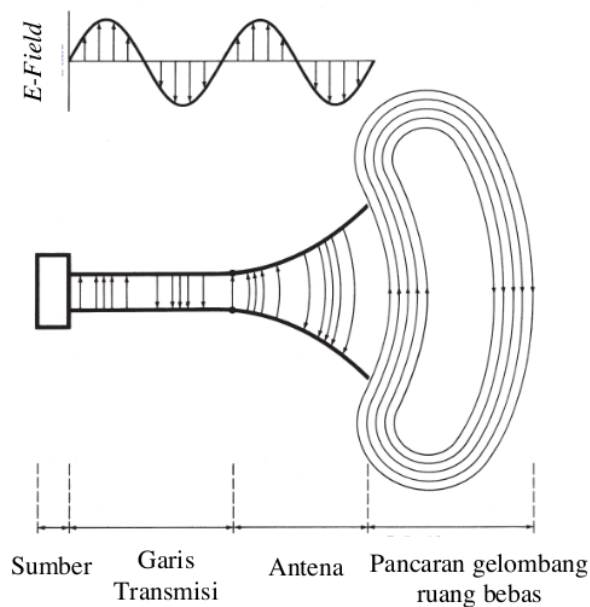
Gambar 2.1 Antena Sebagai Perangkat Transisi [17]
