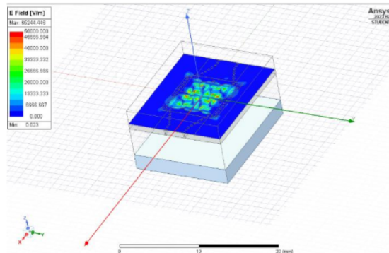
Gambar 4.21 Hasil Simulasi Radiasi dengan Timbal Tiga Lapis
