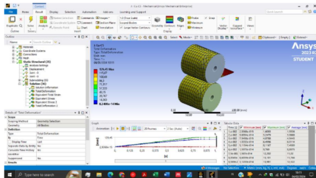
Gambar B.8 Hasil Simulasi Pencanaian Tembaga Tiga Lapis
