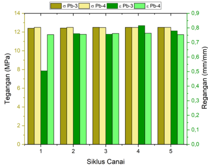
Gambar 4.17 Grafik Tegangan-Regangan Pelat Pb 3 Lapis dan 4 Lapis
