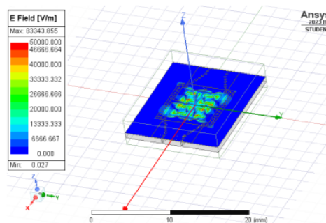
Gambar 4.18 Hasil Simulasi Antena
