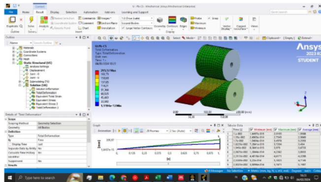
Gambar B.12 Hasil Simulasi Pencanaian Timbal Empat Lapis
