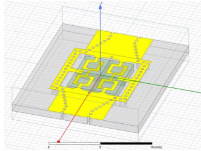
Gambar 3.3 Desain Antena SIW Aperture 5G [58]
