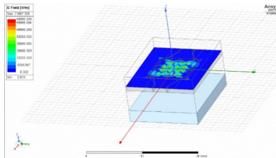
Gambar 4.24 Hasil Simulasi Radiasi dengan Timbal Empat Lapis
