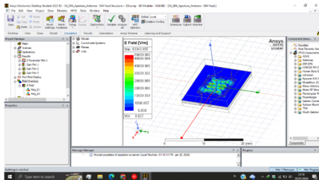
Gambar B.16 Hasil Simulasi Radiasi Antena
