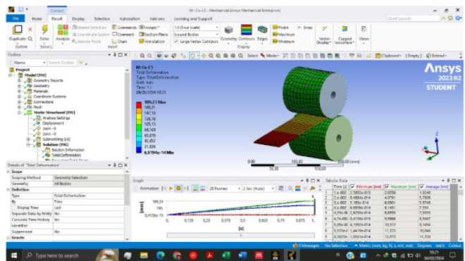
Gambar B.11 Hasil Simulasi Pencanaian Tembaga Empat Lapis
