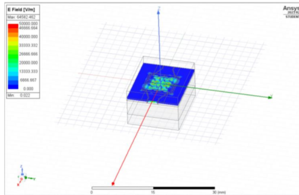
Gambar 4.22 Hasil Simulasi Radiasi dengan Aluminium Empat Lapis
