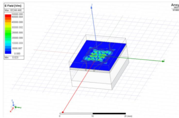
Gambar 4.19 Hasil Simulasi Radiasi dengan Aluminium Tiga Lapis
