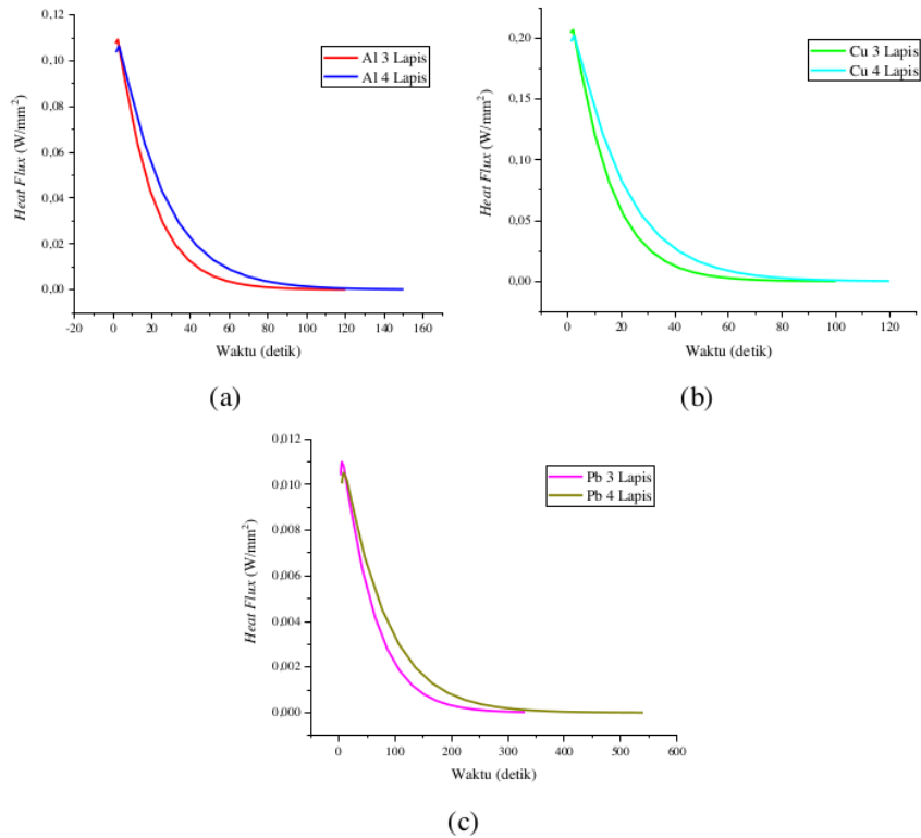
Gambar 4.5 Kurva Waktu Terhadap Heat Flux pada Pelat Tiga dan Empat Lapis pada Al (a), Cu (b), dan Pb (c)
