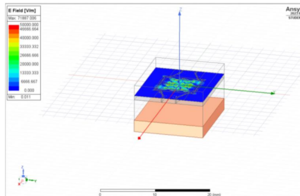
Gambar 4.23 Hasil Simulasi Radiasi dengan Tembaga Empat Lapis
