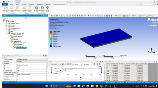
Gambar B.6 Hasil Simulasi Pemanasan Timbal Empat Lapis
