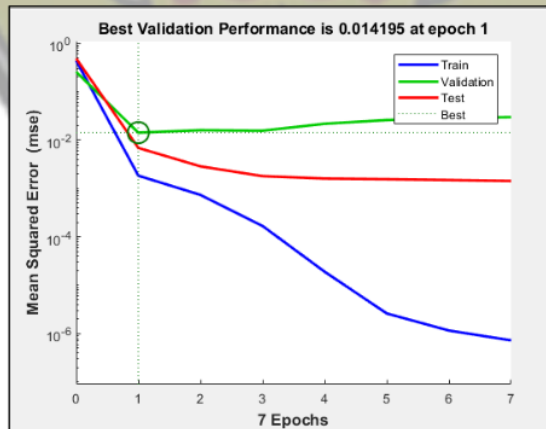
Gambar 16. Grafik Performansi 15 Hidden Layer
