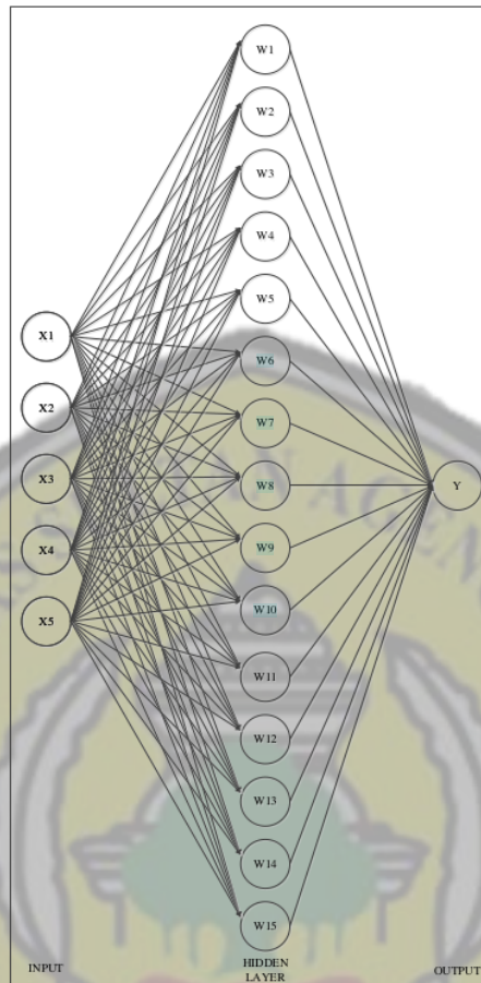
Gambar 8. Arsitektur ANN dengan 15 Hidden Layer
