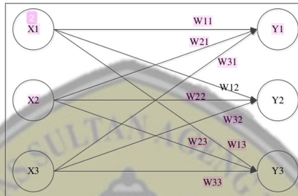
Gambar 1. Arsitektur Jaringan Layer Tunggal
