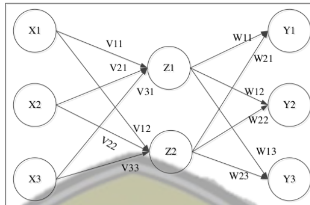
Gambar 2. Arsitektur Jaringan Layer Jamak
