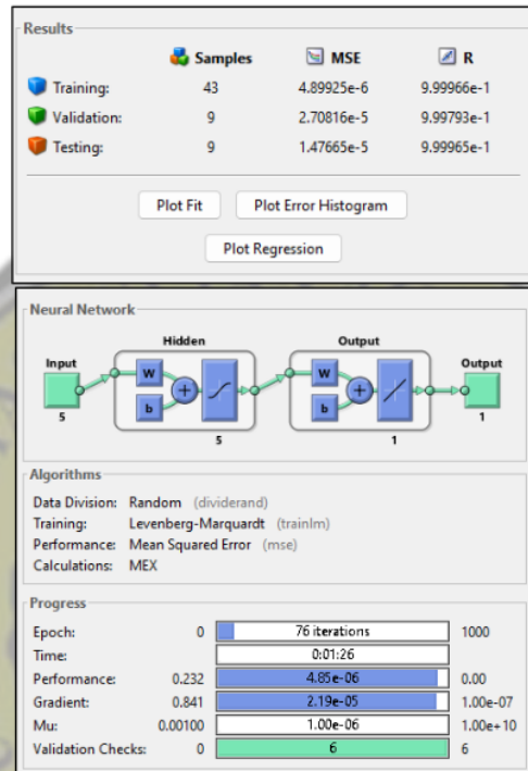
Gambar 9. Hasil Training Data dengan 5 Hidden Layer
