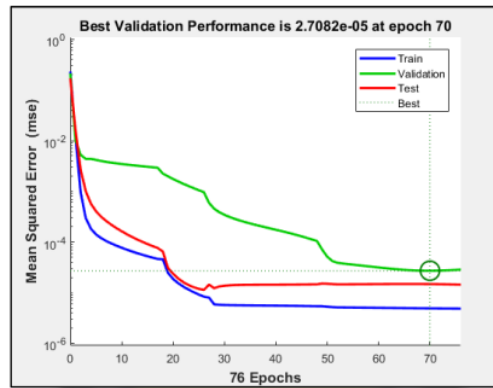
Gambar 10. Grafik Performansi 5 Hidden Layer
