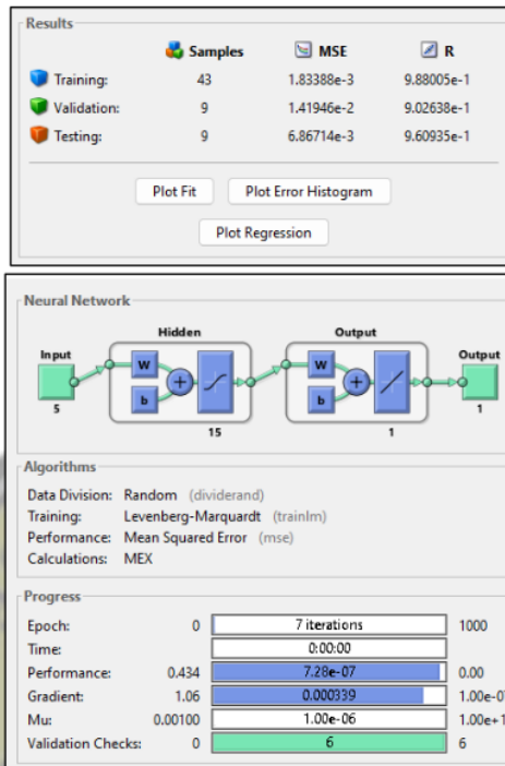
Gambar 15. Hasil Training Data dengan 15 Hidden Layer
