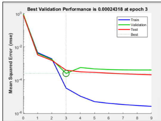
Gambar 13. Grafik Performansi 10 Hidden Layer
