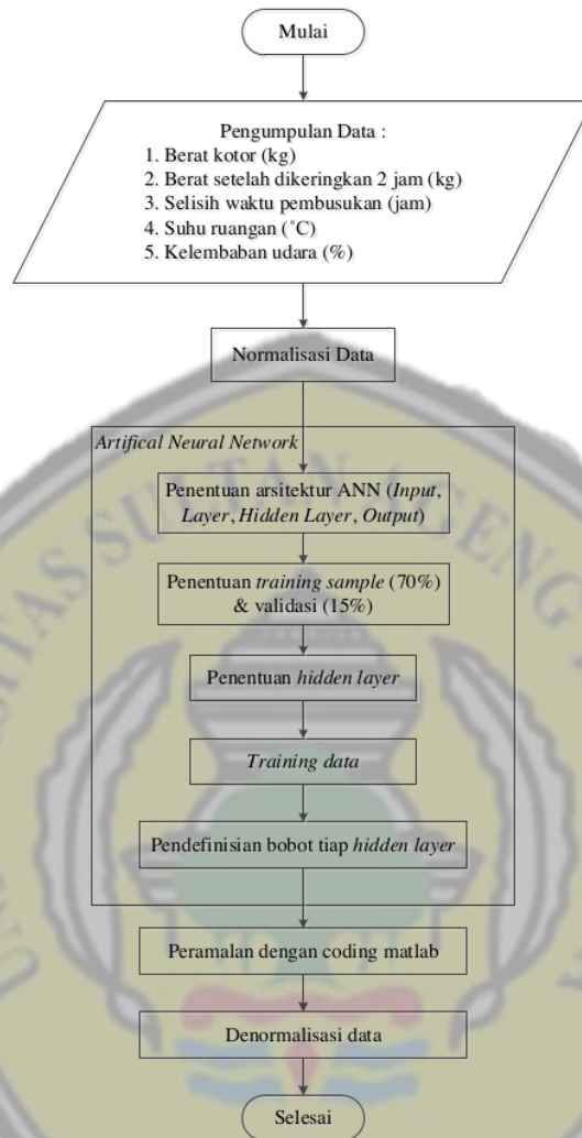
Gambar 4. Flowchart Penyelesaian Masalah
