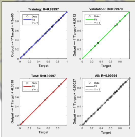
Gambar 11. Grafik Uji Validasi Hasil Training 5 Hidden Layer
