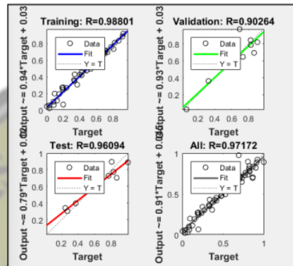
Gambar 17. Grafik Uji Validasi Hasil Training 15 Hidden Layer
