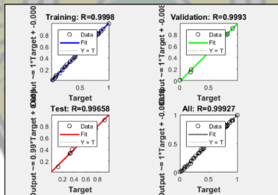
Gambar 14. Grafik Uji Validasi Hasil Training 10 Hidden Layer
