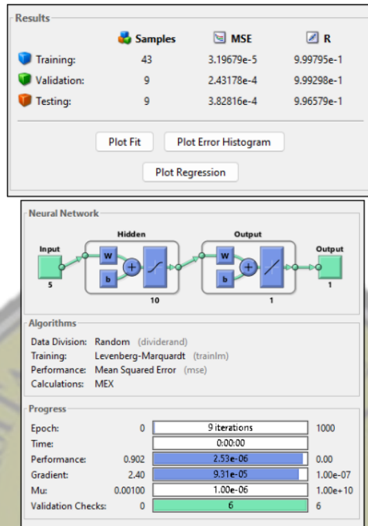
Gambar 12. Hasil Training Data dengan 10 Hidden layer
