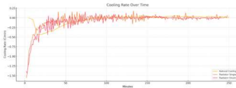
Gambar 4.2 Grafik Laju Pendinginan Terhadap Waktu
