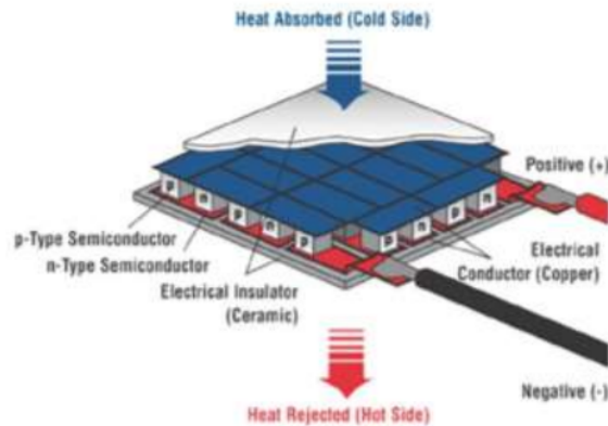
Gambar 2.2 Peltier (termoelektrik)
