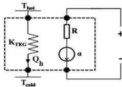
Gambar 2.3 Rangkaian Ekuivalen Peltier (Sumber: Rizaldi & Edahwati, 2022)
