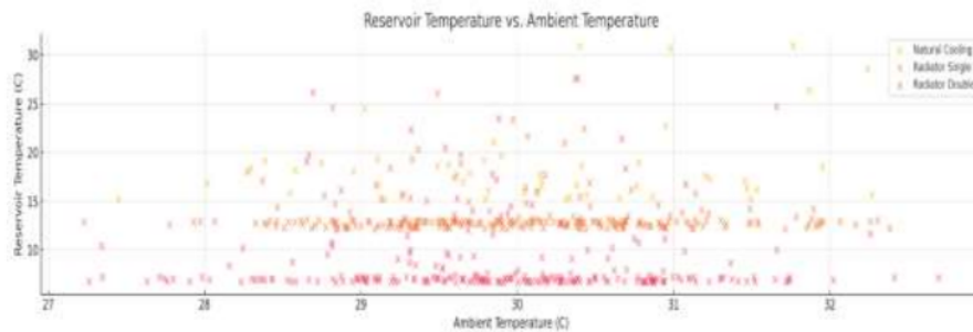
Gambar 4.3 Grafik Plot Sebar reservoir Dari 3 Metode Pendinginan
