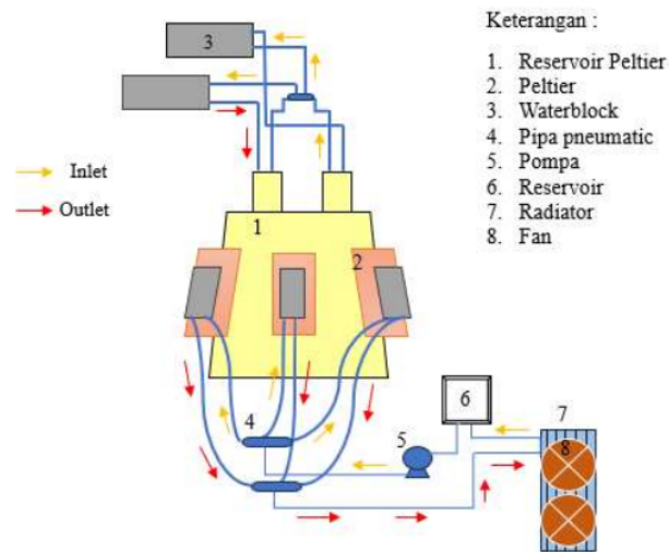
Gambar 2.1 Skema Mesin Kompres Aktif
