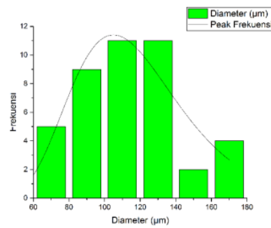
Gambar 4.15 Histogram SEM PUR-21
