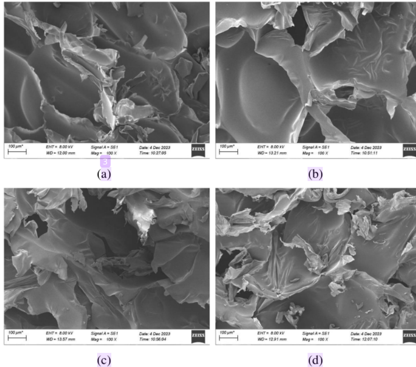
Gambar 4.13 Hasil Perbesaran Ukuran 100x SEM Busa Poliuretan (a) Sampel PUR-11 (b) Sampel PUR-21 (c) Sampel PUR-22 dan (d) Sampel PUR-23
