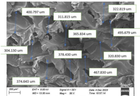
Gambar B.11 SEM PUR-22 Ukuran 50x
