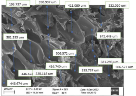
Gambar B.9 SEM PUR-11 Ukuran 50x
