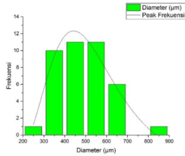
Gambar 4.10 Histogram SEM PUR-21
