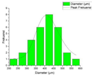
Gambar 4.11 Histogram SEM PUR-22
