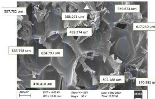
Gambar B.10 SEM PUR-21 Ukuran 50x
