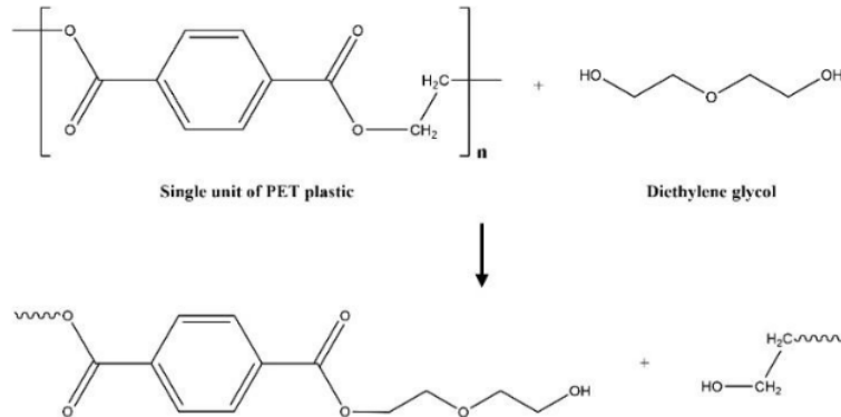
Gambar 2.5 Reaksi PET Dengan DEG dan Penambahan Katalis [14]
