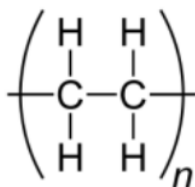
Gambar 2.7 Struktur Kimia HDPE
