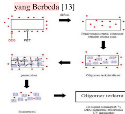
Gambar 2.4 Mekanisme Depolimerisasi PET oleh DEG [14]
