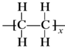
Gambar 2.9 Struktur Kimia LLPE
