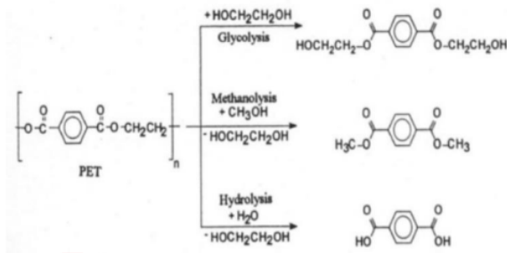
Gambar 2.3 Reaksi Depolimerisasi PET dengan Berbagai Pelarut
