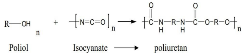
Gambar 2.12 Reaksi Pembuatan Poliuretan [19]
