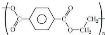
Gambar 2.1 Struktur Kimia PET [8]
