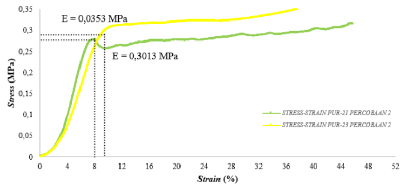
Gambar 4.5 Grafik Stress-Strain Variasi Komposisi Aquades (a) 4,6% Sampel PUR-21 Percobaan 2 dan (b) 1,5% Sampel PUR-23 Percobaan 2
