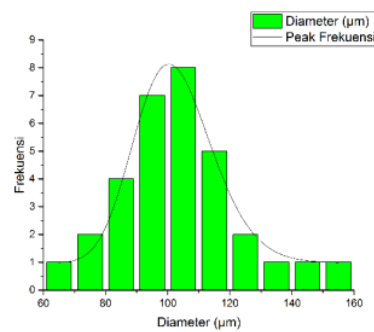
Gambar 4.17 Histogram SEM PUR-23
