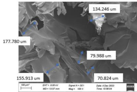
Gambar B.15 SEM PUR-22 Ukuran 50x
