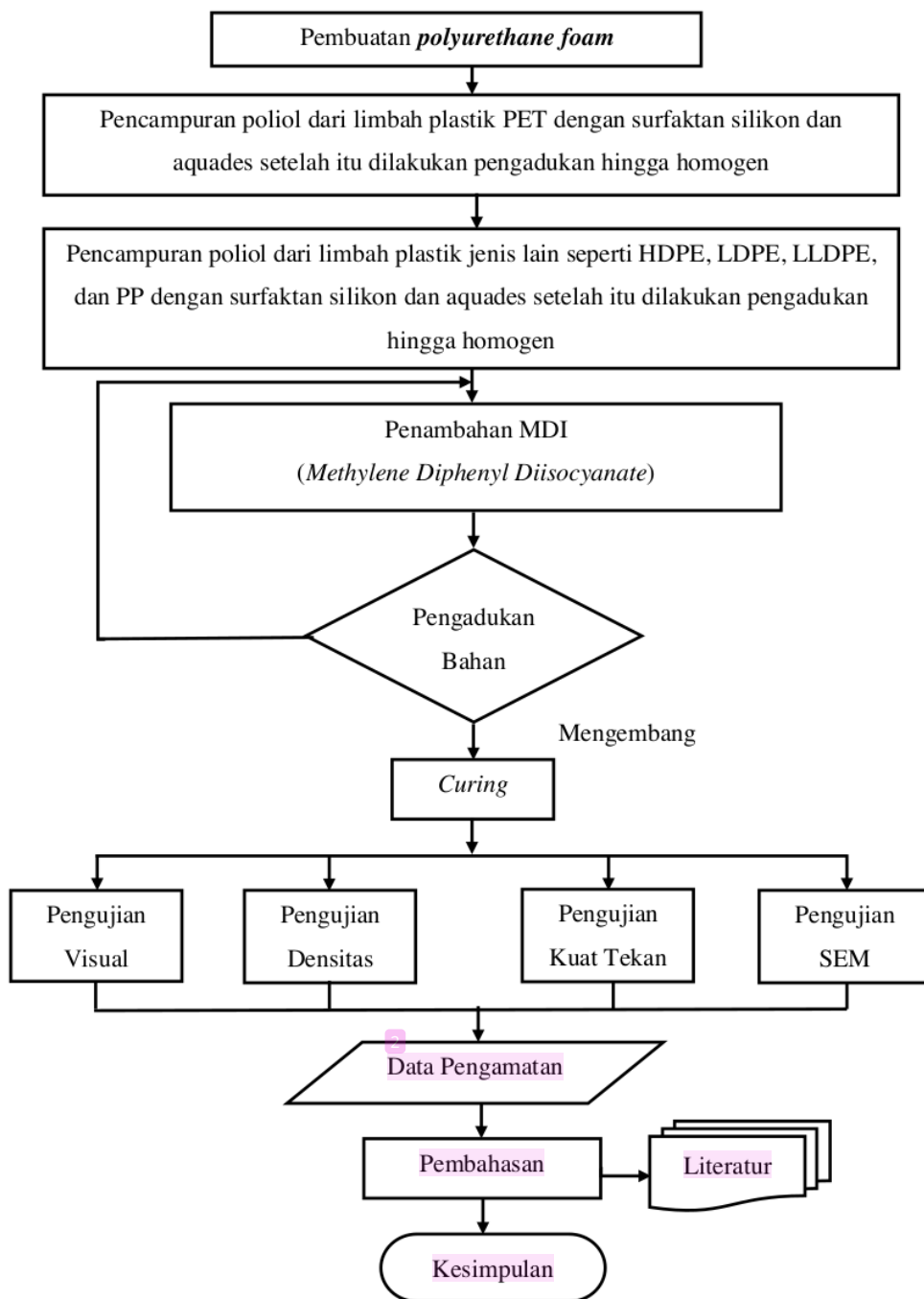
Gambar 3.1 Diagram Alir Pembuatan Busa Poliuretan
