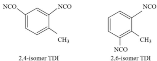
Gambar 2.13 Struktur Toluena Diisosianat (TDI)
