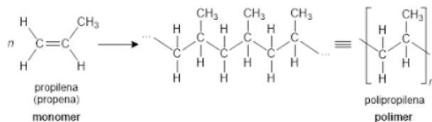
Gambar 2.10 Struktur Kimia PP
