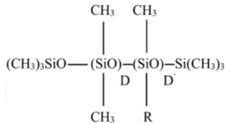
Gambar 2.16 Struktur Surfaktan Silikon pada Busa Poliuretan [21]
