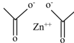
Gambar 2.18 Struktur Zinc Acetate
