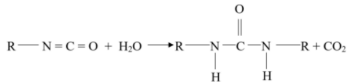
Gambar 2.15 Reaksi Isonianat dengan Air [20]
