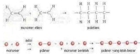
Gambar 2.8 Struktur Kimia LDPE [16]
