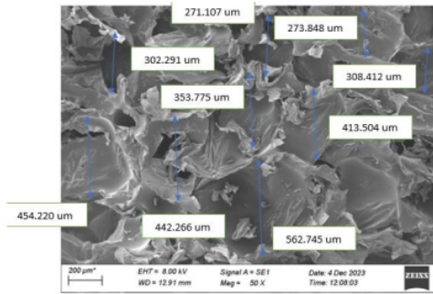
Gambar B.12 SEM PUR-23 Ukuran 50x
