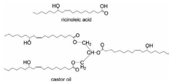
Gambar 2.2 Struktur Kimia Castor Oil dan Asam Ricinoleat [15]
