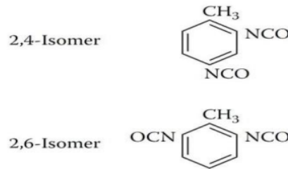
Gambar 2.5 Struktur Kimia TDI [17]
