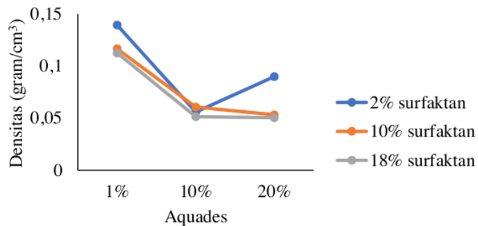
Gambar 4.4 Pengaruh Penambahan Variasi Komposisi Aquades Terhadap Densitas Busa Poliuretan
