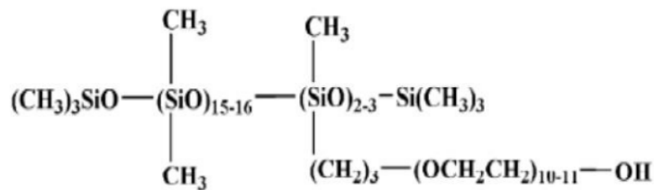
Gambar 2.8 Struktur Kimia Surfaktan Silikon [30]
