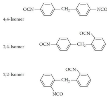
Gambar 2.6 Struktur Kimia MDI [17]
