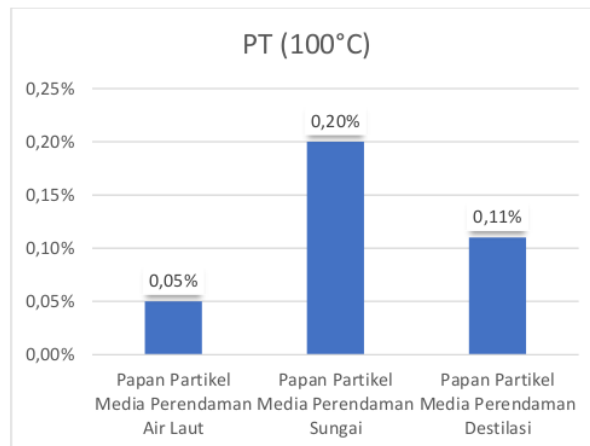
Gambar 4. 3 Grafik Presentase Penyusutan Tebal Papan Partikel di Suhu 100°C
