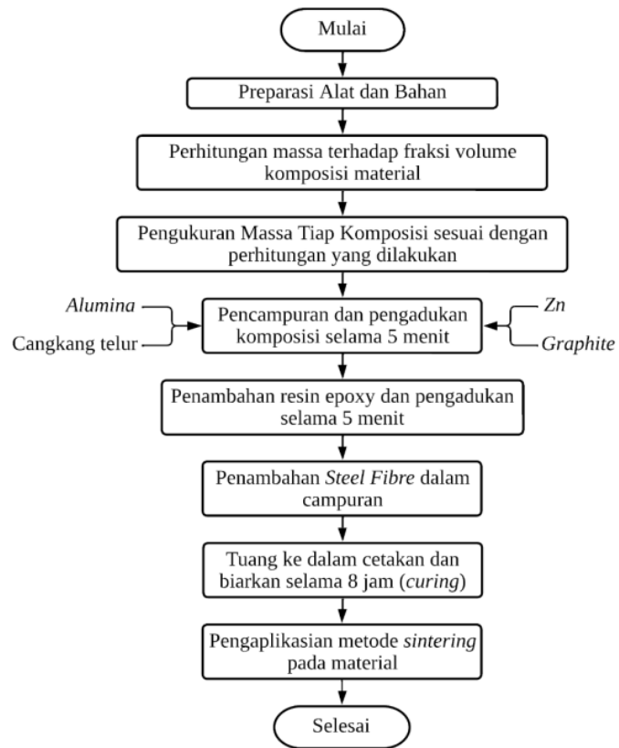
Gambar 3. 13 Diagram Pembuatan Komposit
