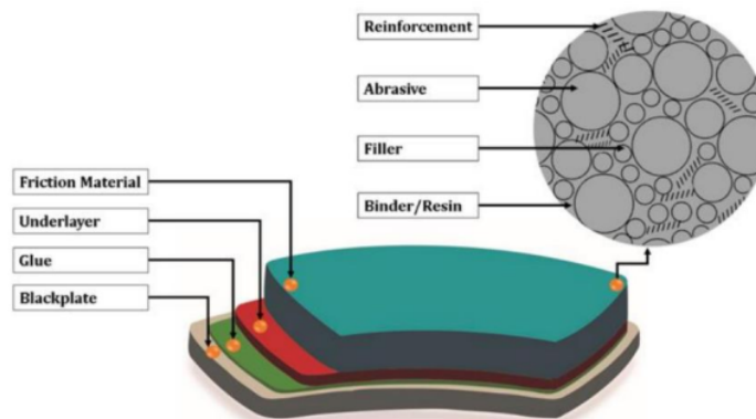
Gambar 2.2 Bagian pada Kampas Rem
