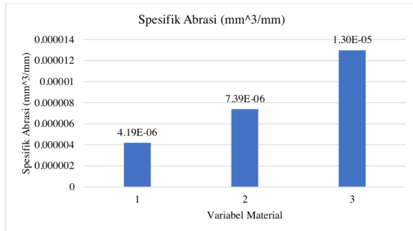
Gambar 4.3 Grafik Uji Keausan
