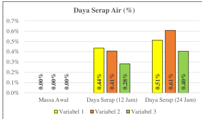
Gambar 4.4 Grafik Daya Serap Air
