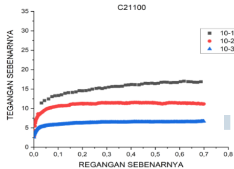
Gambar 4.5 Grafik Hasil Hot Compression Test Pada Spesimen C2 Dengan Temperatur 1100 °C Pada Strain Rate (a) 10^{-1} \text{ s}^{-1} (b) 10^{-2} \text{ s}^{-1} (c) 10^{-3} \text{ s}^{-1}
