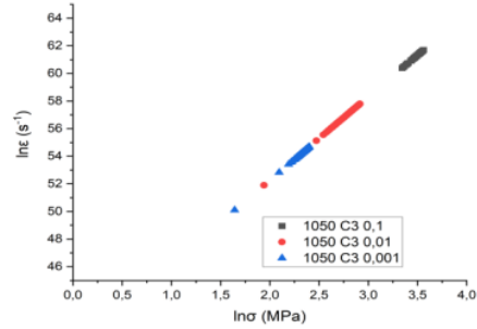
Gambar 4.10 Grafik \ln \sigma vs \ln \epsilon Pada Spesimen C3 Dengan Temperatur 1050\text{ }^{\circ}\text{C} Pada Strain Rate (a) 10^{-1}\text{ s}^{-1} (b) 10^{-2}\text{ s}^{-1} (c) 10^{-3}\text{ s}^{-1}
