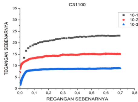
Gambar 4.6 Grafik Hasil Hot Compression Test Pada Spesimen C3 Dengan Temperatur 1100 °C Pada Strain Rate (a) 10^{-1} \text{ s}^{-1} (b) 10^{-2} \text{ s}^{-1} (c) 10^{-3} \text{ s}^{-1}
