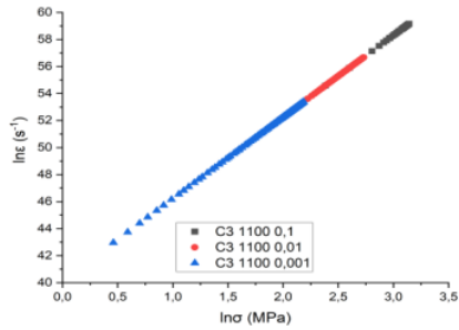
Gambar 4.13 Grafik \ln\sigma vs \ln\epsilon Pada Spesimen C3 Dengan Temperatur 1100\text{ }^{\circ}\text{C} Pada Strain Rate (a) 10^{-1}\text{ s}^{-1} (b) 10^{-2}\text{ s}^{-1} (c) 10^{-3}\text{ s}^{-1}
