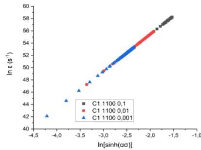
Gambar 4.23 Grafik \ln[\sinh(\alpha\sigma)] vs \ln\epsilon Pada Spesimen C1 Dengan Temperatur 1100 °C Pada Strain Rate (a) 10^{-1} \text{ s}^{-1} (b) 10^{-2} \text{ s}^{-1} (c) 10^{-3} \text{ s}^{-1}
