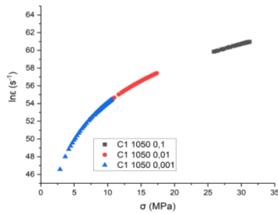
Gambar 4.14 Grafik \sigma vs \ln\epsilon Pada Spesimen C1 Dengan Temperatur 1050\text{ }^{\circ}\text{C} Pada Strain Rate (a) 10^{-1}\text{ s}^{-1} (b) 10^{-2}\text{ s}^{-1} (c) 10^{-3}\text{ s}^{-1}
