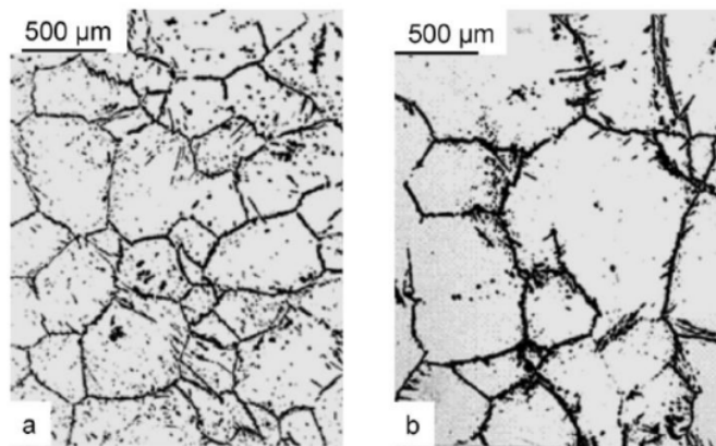
Gambar 2.5 Struktur Mikro Sampel Pengujian Metalografi Pada 1100°C (a) dan 1050°C (b) (Akta et al., 2005)
