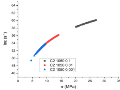
Gambar 4.15 Grafik \sigma vs \ln\epsilon Pada Spesimen C2 Dengan Temperatur 1050\text{ }^{\circ}\text{C} Pada Strain Rate (a) 10^{-1}\text{ s}^{-1} (b) 10^{-2}\text{ s}^{-1} (c) 10^{-3}\text{ s}^{-1}
