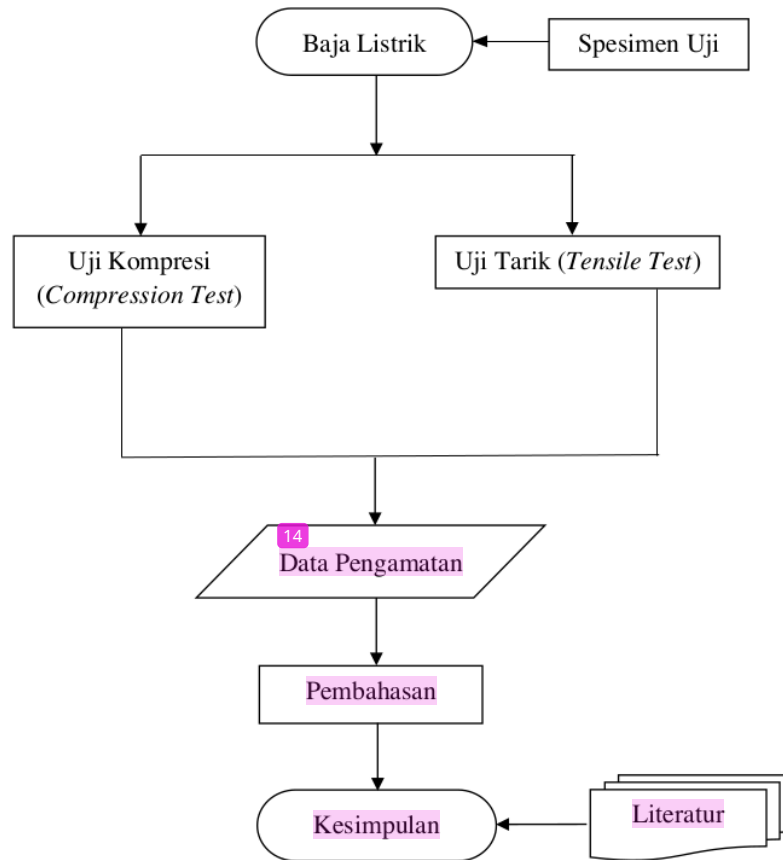
Gambar 3.1 Diagram Alir Percobaan
