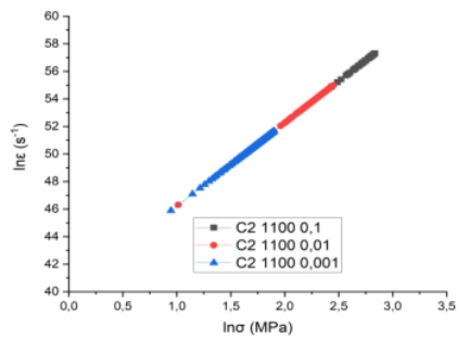
Gambar 4.12 Grafik \ln \sigma vs \ln \epsilon Pada Spesimen C2 Dengan Temperatur 1100\text{ }^{\circ}\text{C} Pada Strain Rate (a) 10^{-1}\text{ s}^{-1} (b) 10^{-2}\text{ s}^{-1} (c) 10^{-3}\text{ s}^{-1}
