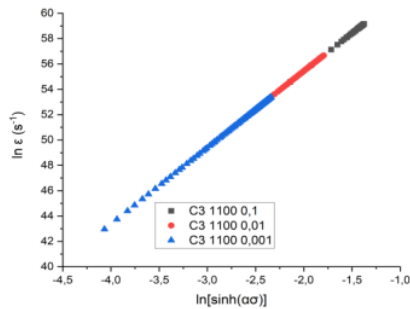
Gambar 4.25 Grafik \ln[\sinh(\alpha\sigma)] vs \ln\dot{\epsilon} Pada Spesimen C3 Dengan Temperatur 1100 °C Pada Strain Rate (a) 10^{-1} \text{ s}^{-1} (b) 10^{-2} \text{ s}^{-1} (c) 10^{-3} \text{ s}^{-1}
