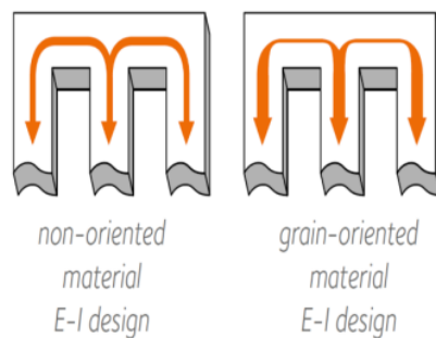
Gambar 2.3 Desain E-I Pada 2 Jenis Baja Listrik (Dough, 2019)
