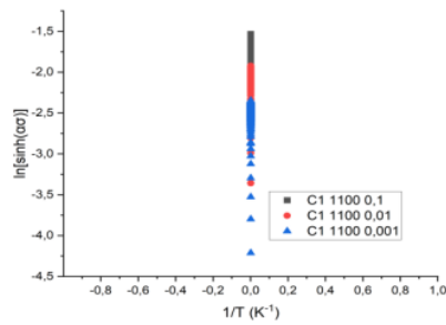
Gambar 4.29 Grafik \frac{1}{T} vs \ln[\sinh(\alpha\sigma)] Pada Spesimen C1 Dengan Temperatur 1100 °C Pada Strain Rate (a) 10^{-1} \text{ s}^{-1} (b) 10^{-2} \text{ s}^{-1} (c) 10^{-3} \text{ s}^{-1}
