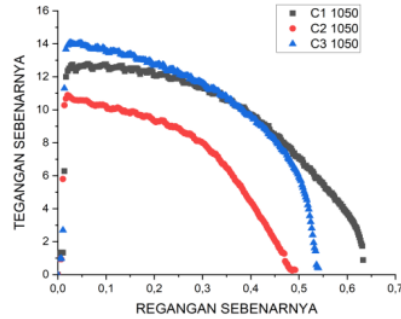
Gambar 4.32 Grafik Hasil Hot Tensile Test Pada Temperatur 1050 °C Pada Spesimen (a) C1 (b) C2 (c) C3
