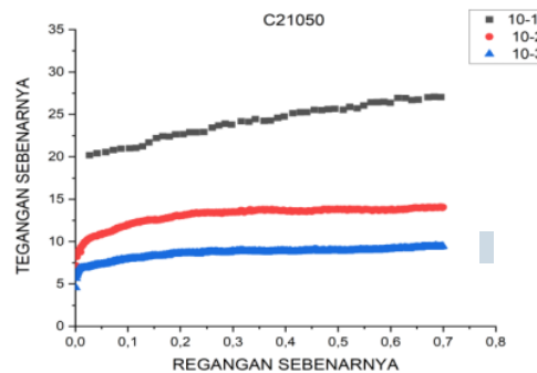
Gambar 4.2 Grafik Hasil Hot Compression Test Pada Spesimen C2 Dengan Temperatur 1050 °C Pada Strain Rate (a) 10^{-1} \text{ s}^{-1} (b) 10^{-2} \text{ s}^{-1} (c) 10^{-3} \text{ s}^{-1}
