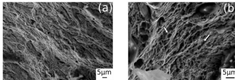
Gambar 2.8 Struktur Mikro Sampel Pengujian Fraktografi Pada 1100°C (a) dan 1050°C (b) (Franceschi et al., 2020)
