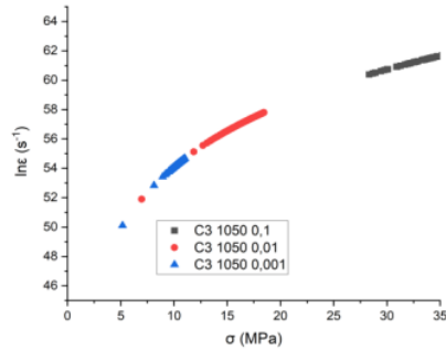
Gambar 4.16 Grafik \sigma vs \ln \epsilon Pada Spesimen C3 Dengan Temperatur 1050 °C Pada Strain Rate (a) 10^{-1} \text{ s}^{-1} (b) 10^{-2} \text{ s}^{-1} (c) 10^{-3} \text{ s}^{-1}
