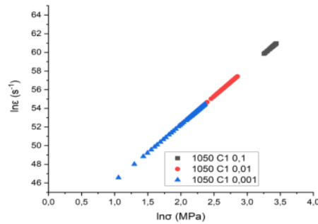
Gambar 4.8 Grafik \ln \sigma vs \ln \epsilon Pada Spesimen C1 Dengan Temperatur 1050 \text{ }^{\circ}\text{C} Pada Strain Rate (a) 10^{-1} \text{ s}^{-1} (b) 10^{-2} \text{ s}^{-1} (c) 10^{-3} \text{ s}^{-1}
