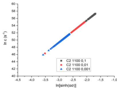
Gambar 4.24 Grafik \ln[\sinh(\alpha\sigma)] vs \ln\epsilon Pada Spesimen C2 Dengan Temperatur 1100 °C Pada Strain Rate (a) 10^{-1} \text{ s}^{-1} (b) 10^{-2} \text{ s}^{-1} (c) 10^{-3} \text{ s}^{-1}
