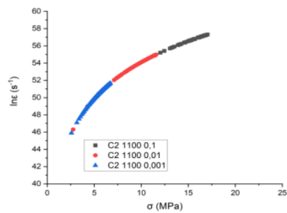
Gambar 4.18 Grafik \sigma vs \ln \epsilon Pada Spesimen C2 Dengan Temperatur 1100 °C Pada Strain Rate (a) 10^{-1} \text{ s}^{-1} (b) 10^{-2} \text{ s}^{-1} (c) 10^{-3} \text{ s}^{-1}
