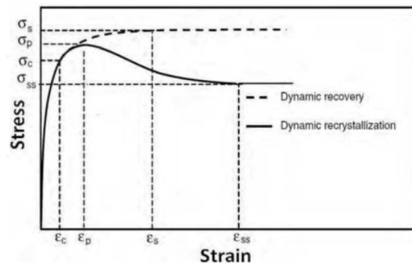
Gambar 4.7 Skema Grafik DRV dan DRX
