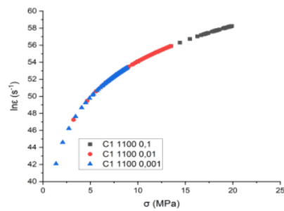
Gambar 4.17 Grafik \sigma vs \ln \epsilon Pada Spesimen C1 Dengan Temperatur 1100 °C Pada Strain Rate (a) 10^{-1} \text{ s}^{-1} (b) 10^{-2} \text{ s}^{-1} (c) 10^{-3} \text{ s}^{-1}
