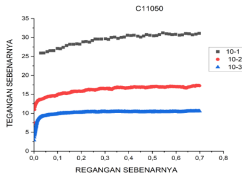
Gambar 4.1 Grafik Hasil Hot Compression Test Pada Spesimen C1 Dengan Temperatur 1050 °C Pada Strain Rate (a) 10^{-1} \text{ s}^{-1} (b) 10^{-2} \text{ s}^{-1} (c) 10^{-3} \text{ s}^{-1}
