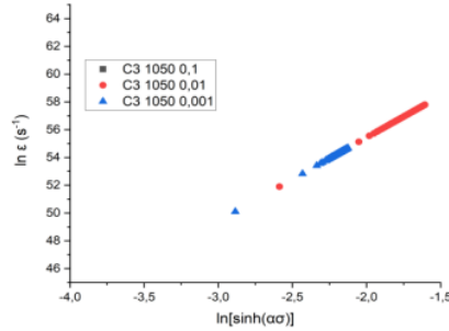
Gambar 4.22 Grafik \ln[\sinh(\alpha\sigma)] vs \ln\epsilon Pada Spesimen C3 Dengan Temperatur 1050 °C Pada Strain Rate (a) 10^{-1} \text{ s}^{-1} (b) 10^{-2} \text{ s}^{-1} (c) 10^{-3} \text{ s}^{-1}
