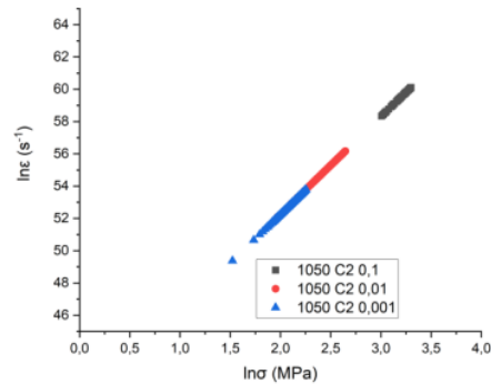
Gambar 4.9 Grafik \ln \sigma vs \ln \epsilon Pada Spesimen C2 Dengan Temperatur 1050 \text{ }^{\circ}\text{C} Pada Strain Rate (a) 10^{-1} \text{ s}^{-1} (b) 10^{-2} \text{ s}^{-1} (c) 10^{-3} \text{ s}^{-1}
