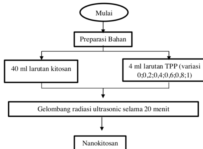
Gambar 3.4 Diagram Alir Pembuatan Nanokitosan
