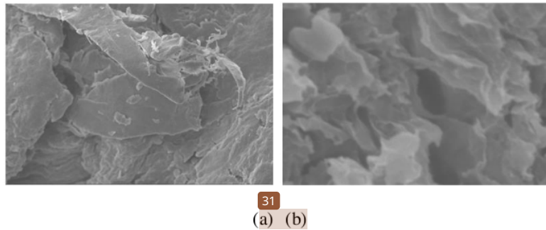
Gambar 4.4 Morfologi Permukaan Hasil SEM Nanokitosan Perbesaran (a) 1000x dan (b) 20.000x
