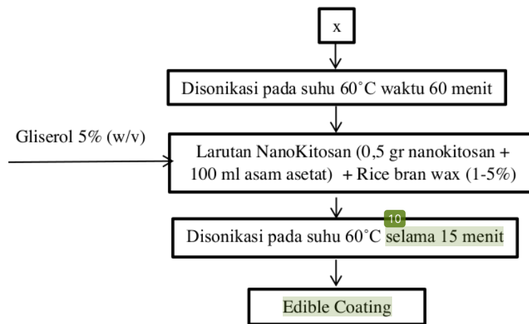
Gambar 3.7 Diagram Alir Pembentukan Edible Coating
