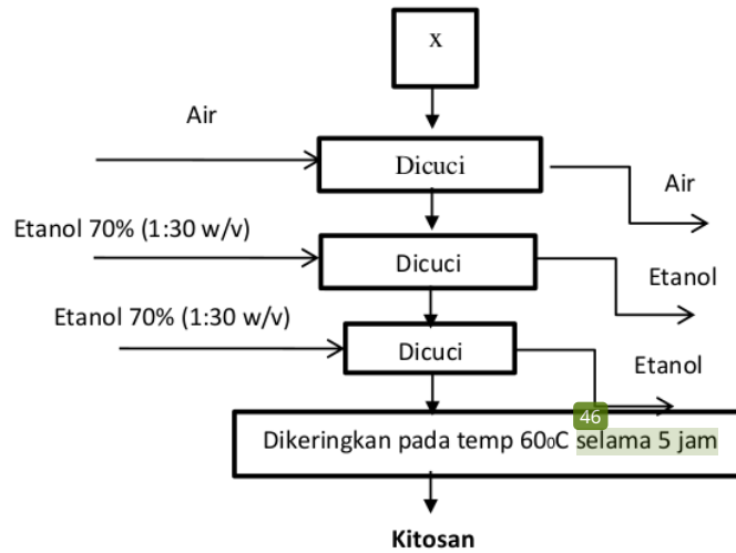
Gambar 3.1 Diagram Alir Pembuatan Kitosan
