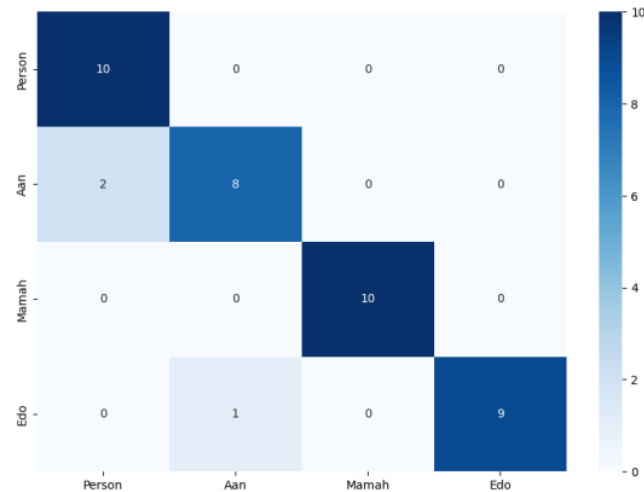
Gambar 4.12 Confusion Matrix Pada Pengujian Kedua
