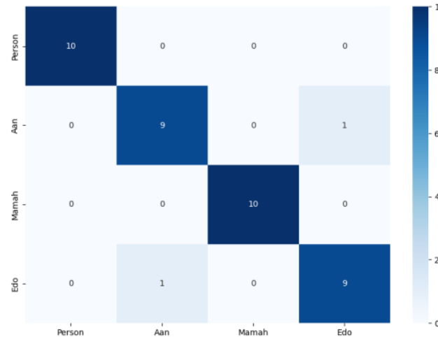
Gambar 4.10 Confusion Matrix Pada Pengujian Pertama
