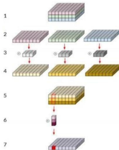
Gambar 2.3 Konvolusi Depthwise dan Pointwise
