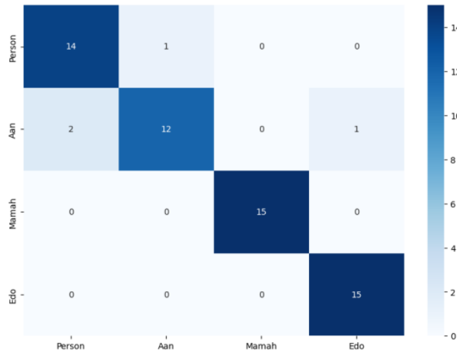
Gambar 4.13 Confusion Matrix Pada Pengujian Kedua
