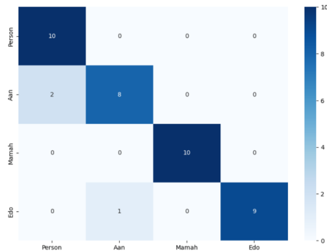
Gambar 4.11 Confusion Matrix Pada Pengujian Pertama
