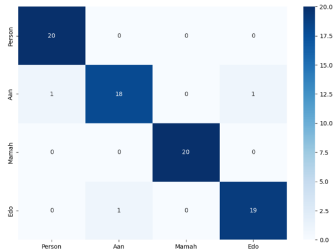
Gambar 4.14 Confusion Matrix Pada Pengujian ketiga
