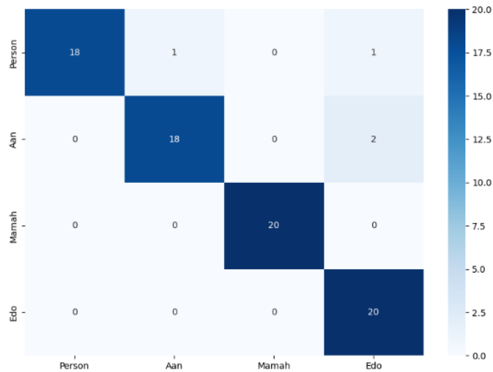
Gambar 4.15 Confusion Matrix Pada Pengujian ketiga
