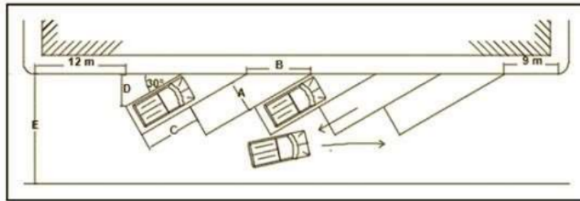
Gambar 3.2 Parkir Menyudut 30°
