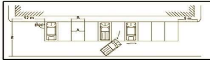
Gambar 3.5 Parkir Membentuk sudut 90°
