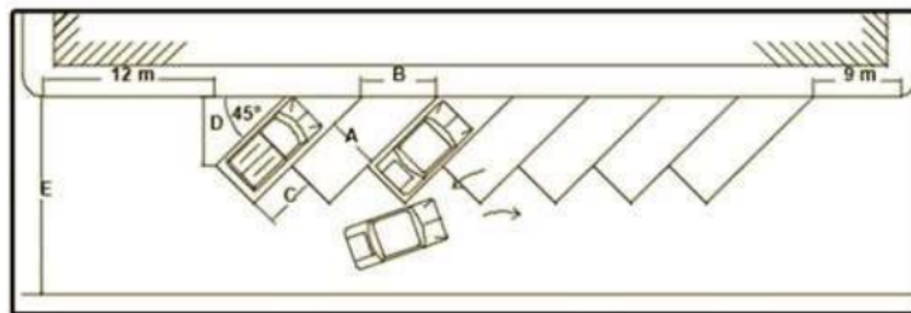
Gambar 3.3 Parkir membentuk sudut 45°
