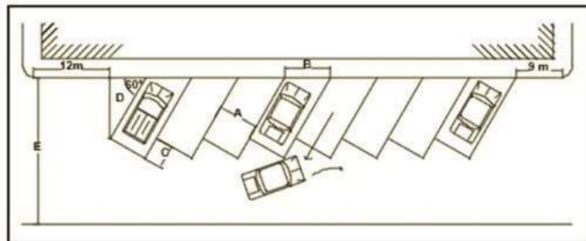
Gambar 3.4 Parkir membentuk sudut 60°
