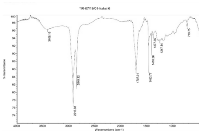
Gambar 2. Spektrum Inframerah (IR) Fraksi 6
