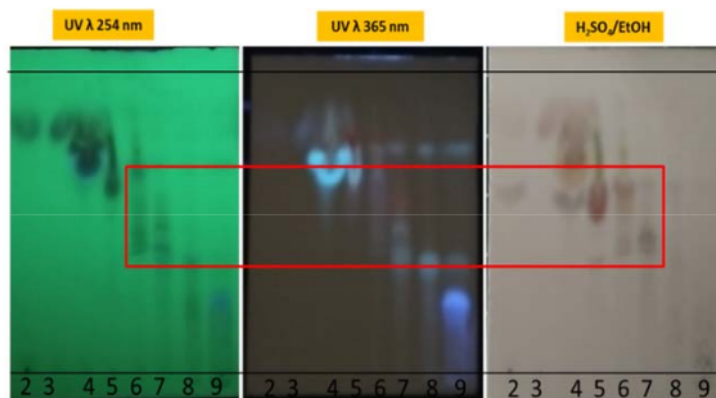
Gambar 1. Hasil KLT Fraksi 2-9.
