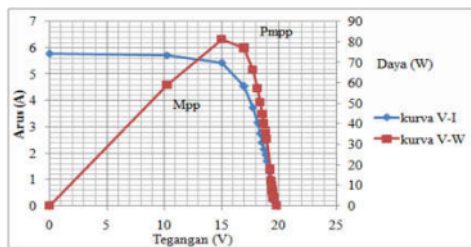
Gambar 7. Kurva P_{MPP}
