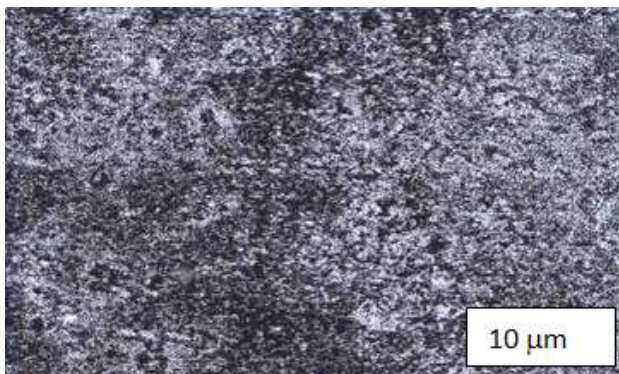
Gambar 4.1. Foto Stuktur Mikro Sampel A 600°C. 500X.
