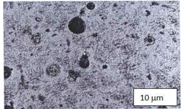
Gambar 4.2. Foto Struktur Mikro Sampel B 600°C. 500X
