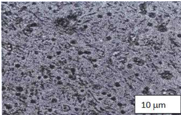
Gambar 4.5. Struktur Mikro Sampel D 600°C.500X
