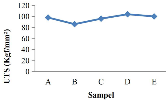
Grafik 4.1. Nilai Kekuatan Tarik Sampel Spheroid Anil
