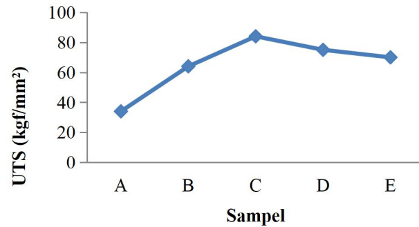
Grafik 4.2. Nilai Kekuatan Tarik Sampel Temper 600°C.
