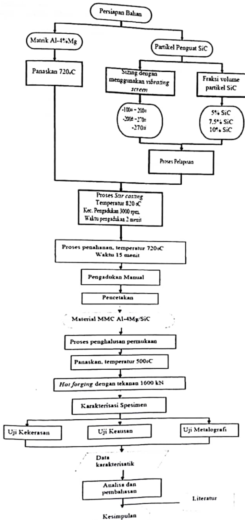
Gambar 5. Diagram alir pembuatan komposit matriks logam paduan Al- 4%Mg/SiC dengan stir casting
