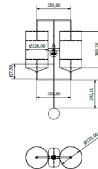
Gambar 2. Dimensi Komponen PLTGL
