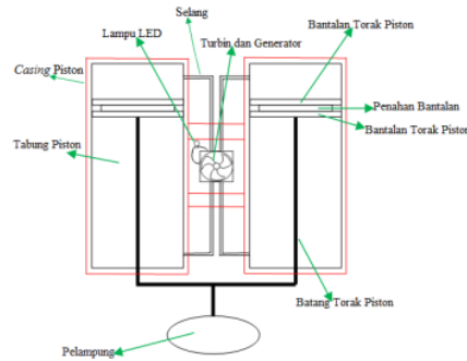
Gambar 1. Komponen dan Rangkaian PLTGL
