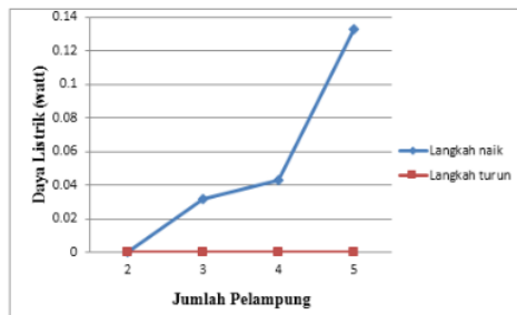
Gambar 3. Grafik Hubungan daya Listrik dan Jumlah Pelampung
