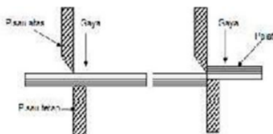
G.1 Prinsip Kerja Pemotongan [3, 7]
