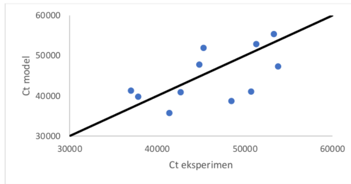
Gambar 2. Plotting antara data eksperimen dengan data terukur
