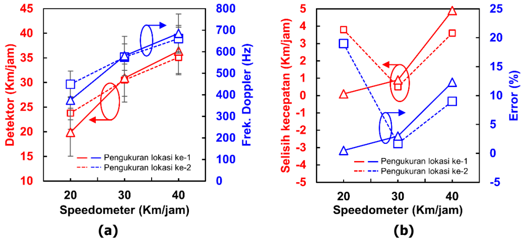
Gambar 9. Hasil pengukuran pada jarak 3 m (a) Perbandingan kecepatan speedometer dengan kecepatan pada detektor serta nilai frekuensi dopplernya, (b) Selisih nilai kecepatan speedometer dan detektor serta nilai kesalahan pembacaannya.
