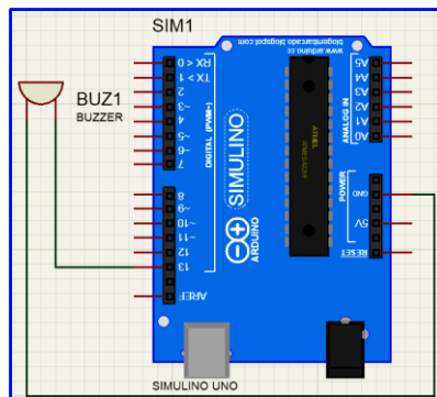
Gambar 5. Skematik Buzzer dan Arduino Uno
