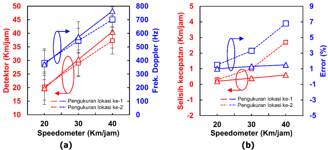
Gambar 12. Hasil pengukuran pada jarak 6 m (a) Perbandingan kecepatan speedometer dengan kecepatan pada detektor serta nilai frekuensi dopplernya, (b) Selisih nilai kecepatan speedometer dan detektor serta nilai kesalahan pembacaannya.
