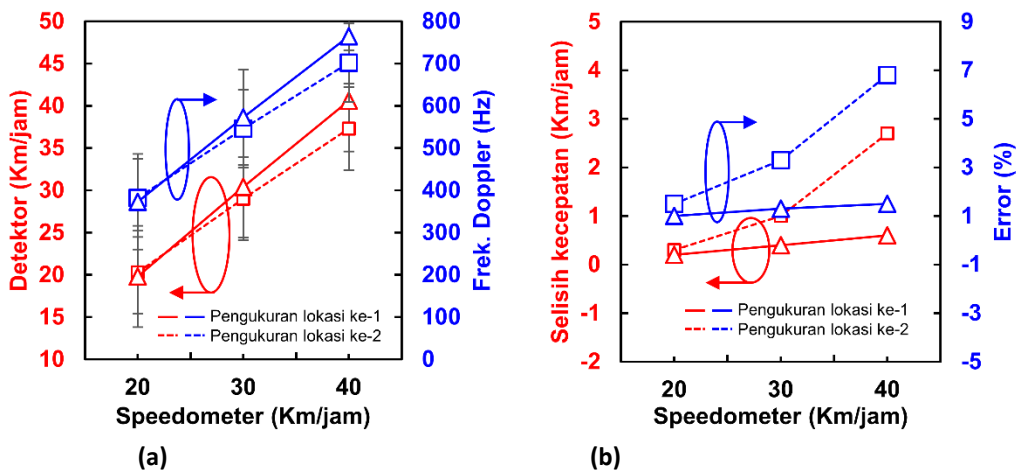
Gambar 12. Hasil pengukuran pada jarak 6 m (a) Perbandingan kecepatan speedometer dengan kecepatan pada detektor serta nilai frekuensi dopplernya, (b) Selisih nilai kecepatan speedometer dan detektor serta nilai kesalahan pembacaannya.
