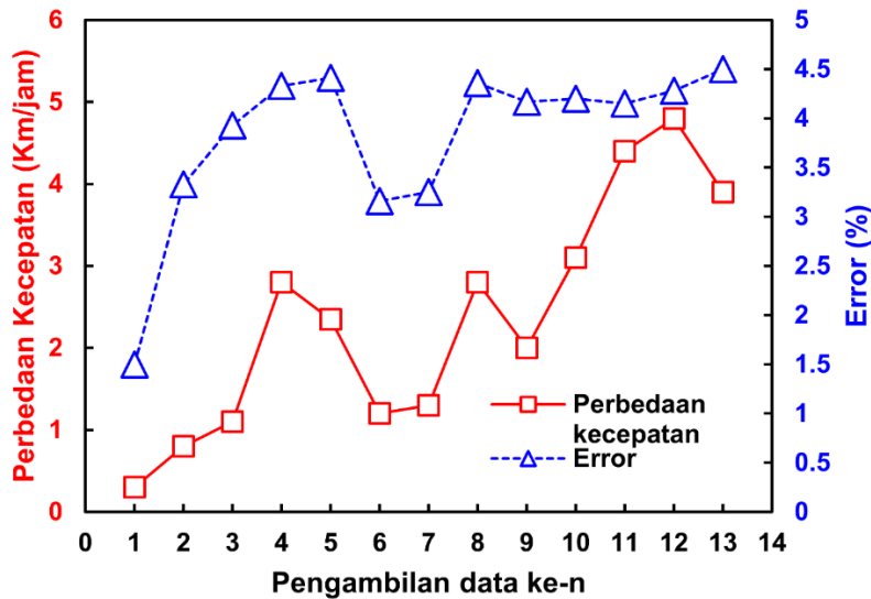
Gambar 14. Perbedaan pengukuran kecepatan menggunakan speedometer dan menggunakan detektor, serta nilai kesalahan deteksi untuk beberapa kali pengambilan data.
