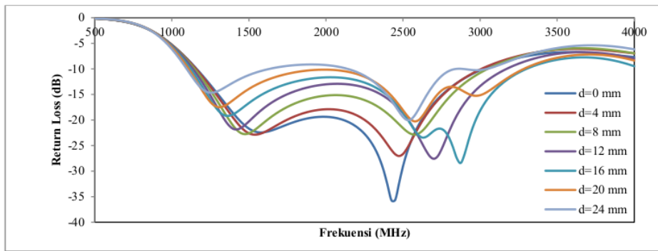
Gambar 5. Proses iterasi nilai d(mm).
