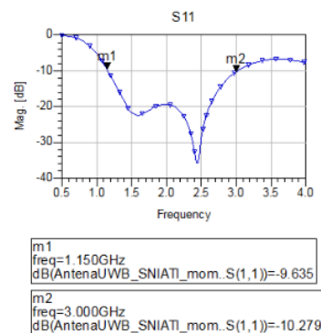
Gambar 2. Simulasi return loss (dB) desain antena mikrostrip lingkaran
