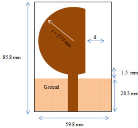
Gambar 3. Desain antena mikrostrip lingkaran dengan beveled half cut
