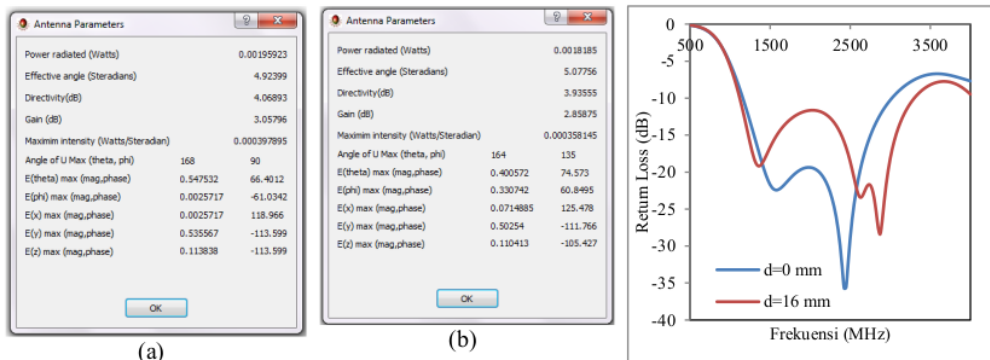
Gambar 6. Perbandingan kinerja antena. (a) Microstrip Lingkaran. (b) Microstrip lingkaran dengan beveled half cut. (c) Perbandingan nilai return loss (dB).
