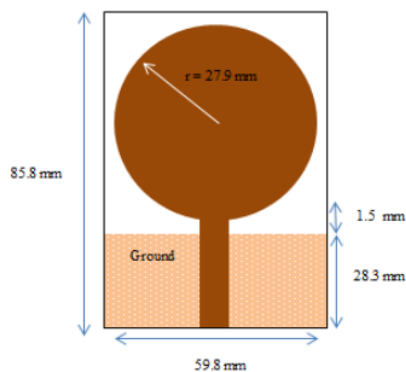
Gambar 1. Desain antena mikrostrip lingkaran
