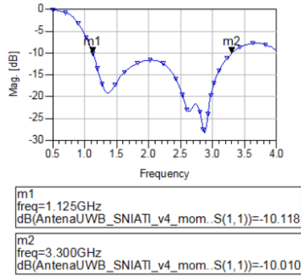
Gambar 4. Simulasi return loss (dB) desain antena mikrostrip lingkaran dengan beveled half cut saat d = 16 mm
