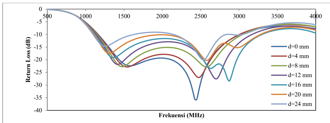
Gambar 5. Proses iterasi nilai d(mm).
