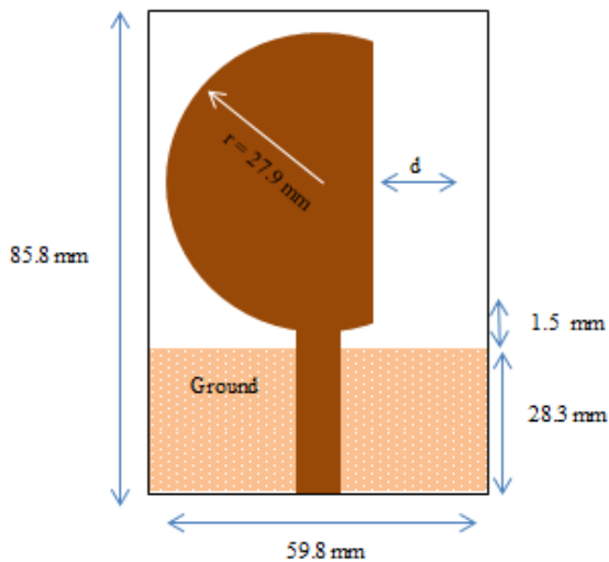
Gambar 3. Desain antena mikrostrip lingkaran dengan beveled half cut
