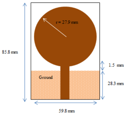
Gambar 1. Desain antena mikrostrip lingkaran
