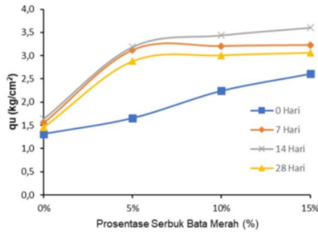
Gambar 7 Grafik hubungan q_u dengan persentase Serbuk Bata Merah
