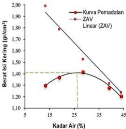
Gambar 6. Grafik Berat Isi Kering terhadap Kadar Air Oprimum
