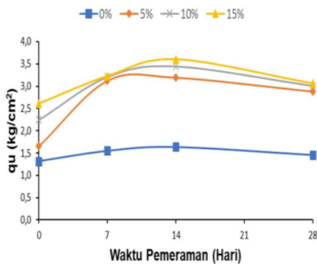
Gambar 8 Grafik Hhubungan q_u terhadap Waktu Pemeraman
