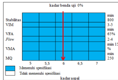
Gambar 9. Grafik Penentuan Optimum dengan Kadar 0%
