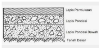
Gambar 1. Lapis perkerasan lentur (Sumber: Silvia Sukirman, 2003)
