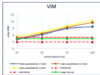
Gambar 4. Grafik Hubungan VIM dan Kadar Disinfektan (Sumber :Analisa Penulis,2021)
