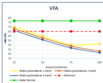
Gambar 5. Grafik Hubungan VFA dan Kadar Disinfektan (Sumber : Analisa Penulis, 2021).
