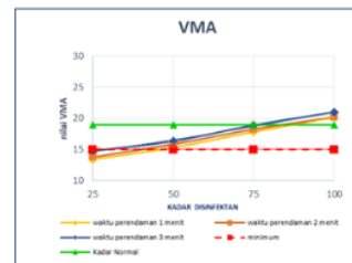
Gambar 3. Grafik Hubungan VMA dan Kadar Disinfektan
