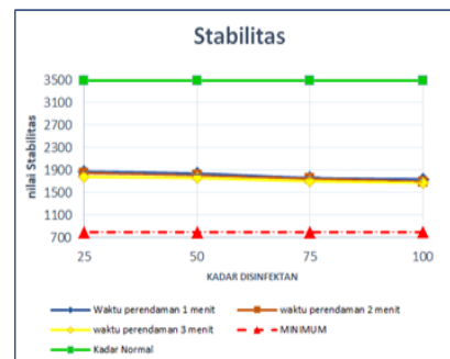
Gambar 6. Grafik Hubungan Stabilitas dan Kadar Disinfektan
