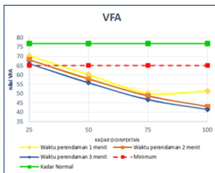
Gambar 5. Grafik Hubungan VFA dan Kadar Disinfektan
