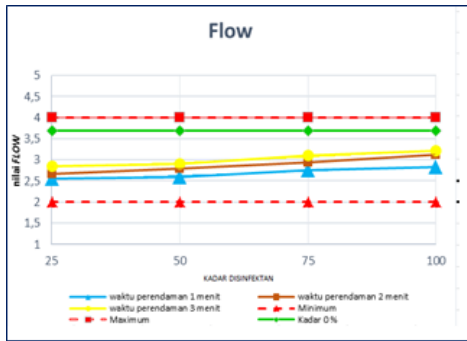
Gambar 7. Grafik Hubungan Flow dan Kadar Disinfektan (Sumber : Analisa Penulis, 2021)
