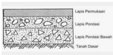
Gambar 1. Lapis perkerasan lentur (Sumber: Silvia Sukirman, 2003)
