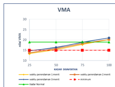
Gambar 3. Grafik Hubungan VMA dan Kadar Disinfektan
