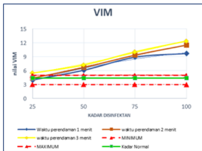
Gambar 4. Grafik Hubungan VIM dan Kadar Disinfektan
