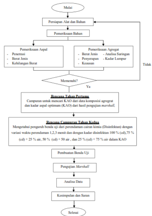
Gambar 2. Diagram Alir Penelitian (Sumber: Dokumen Penulis, 2021)
