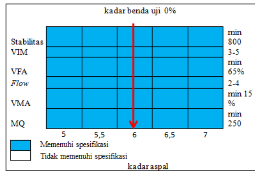
Gambar 9. Grafik Penentuan Optimum dengan Kadar 0%
