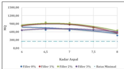
Gambar 7. Perbandingan Nilai MQ
