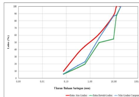
Gambar 1. Gradasi Campuran HRS-WC
