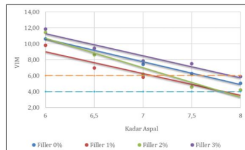
Gambar 3. Perbandingan Nilai VIM
