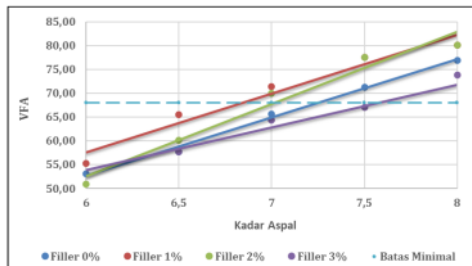
Gambar 4. Perbandingan Nilai VFA
