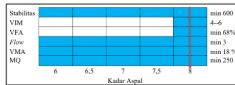
Gambar 11. Penentuan KAO Filler Gypsum 3%
