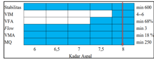
Gambar 8. Penentuan KAO Filler Gypsum 0%
