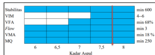
Gambar 10. Penentuan KAO Filler Gypsum 2%
