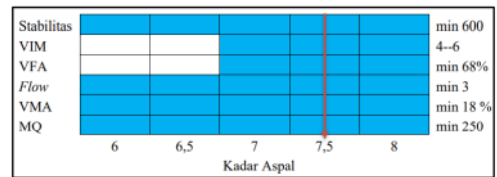
Gambar 9. Penentuan KAO Filler Gypsum 1%
