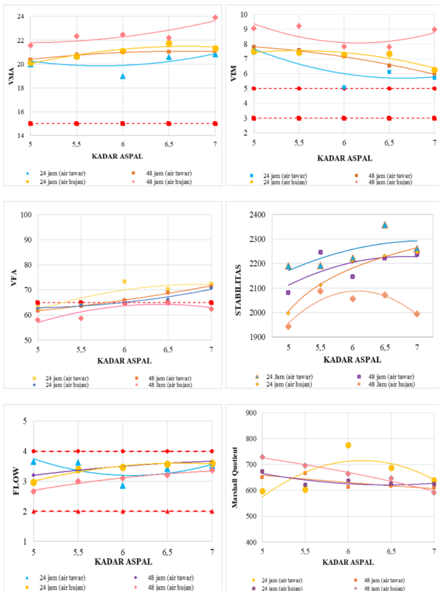
Gambar 2 Hasil Pengujian Marshall
