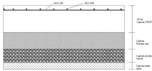
Gambar 4. Potongan Memanjang Perkerasan
