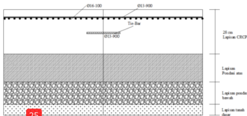
Gambar 3. Potongan Melintang Perkerasan
