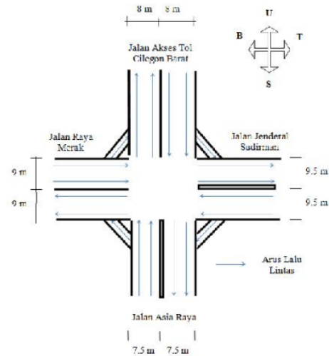
Gambar 2. Denah Simpang Damkar Kondisi existing Sumber : Analisis Penulis, 2013
