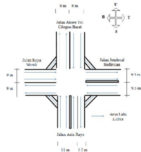
Gambar 3. Denah Simpang Damkar Kondisi saat penerapan contra flow Sumber : Analisis Penulis, 2013
