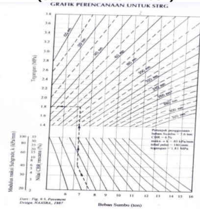
Gambar 7. Grafik Perencanaan Untuk STRG (Sumber : NAASRA 1987)
