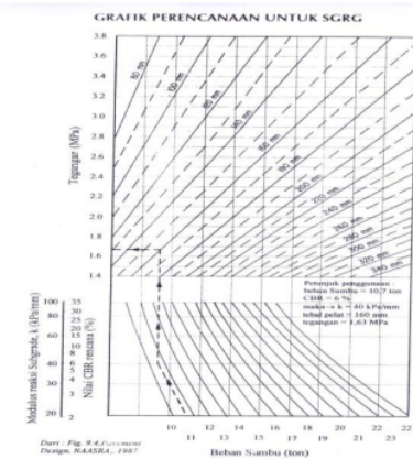
Gambar 8. Grafik Perencanaan Untuk SGRG (Sumber : NAASRA 1987)
