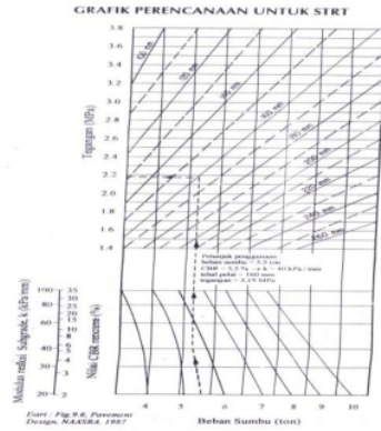
Gambar 6. Grafik Perencanaan Untuk STRT (Sumber : NAASRA 1987)
