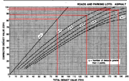
Gambar 5. Kurva CVD
