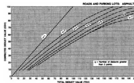
Gambar 2. Kurva hubungan antara TDV, CDV dan q
